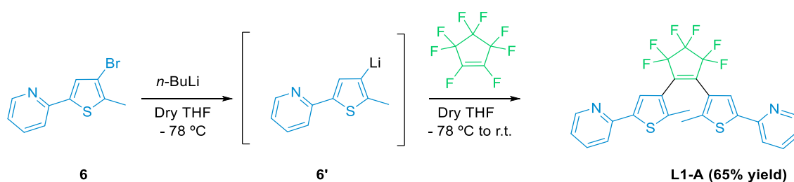
Scheme 2.6. Syntheses of L1-A .
