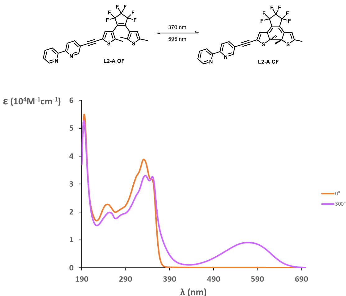
Figure R8. Comportement photochromique (photocyclisation/photocycloversion) pour les ligands DTE synthétisés.
