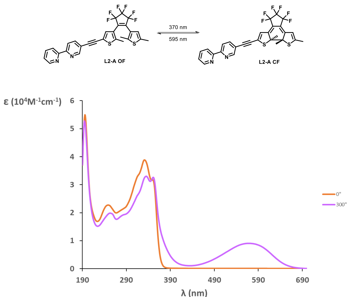
Figura R8. Comportamiento fotocromico (fotociclacion/fotocicloversion) para los ligandos DTE sintetizados.
