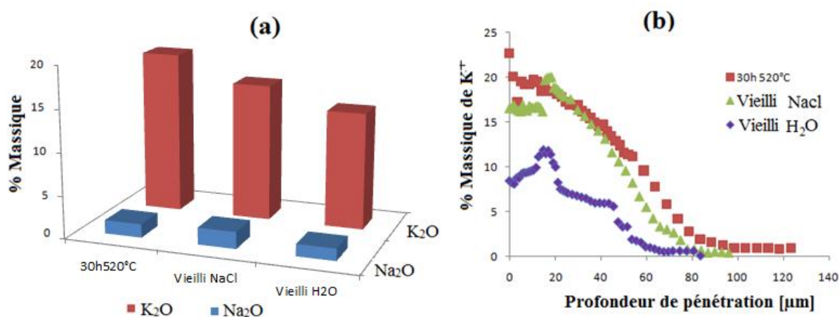
Figure III.17 : (a) Pourcentage massique des ions \text{K}^+ et \text{Na}^+ pour différents états de vieillissement du verre traité. (b) Pourcentage massique d'oxyde de potassium en fonction de la profondeur de pénétration pour différents états de vieillissement.
