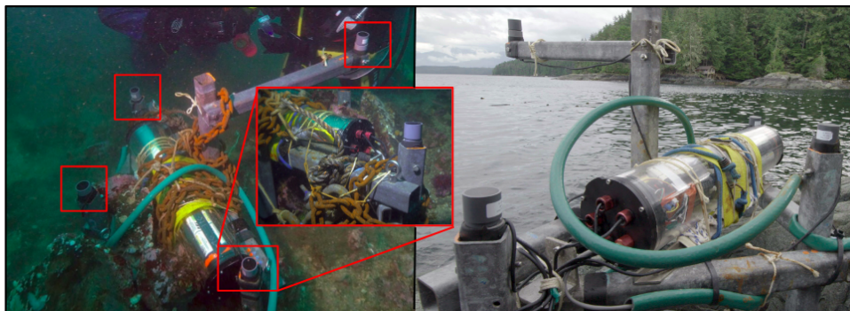
FIG. 2.16 – L'antenne à quatre hydrophones, avec le câble 12 V (vert) connecté à la station de recherche Orcalab.
