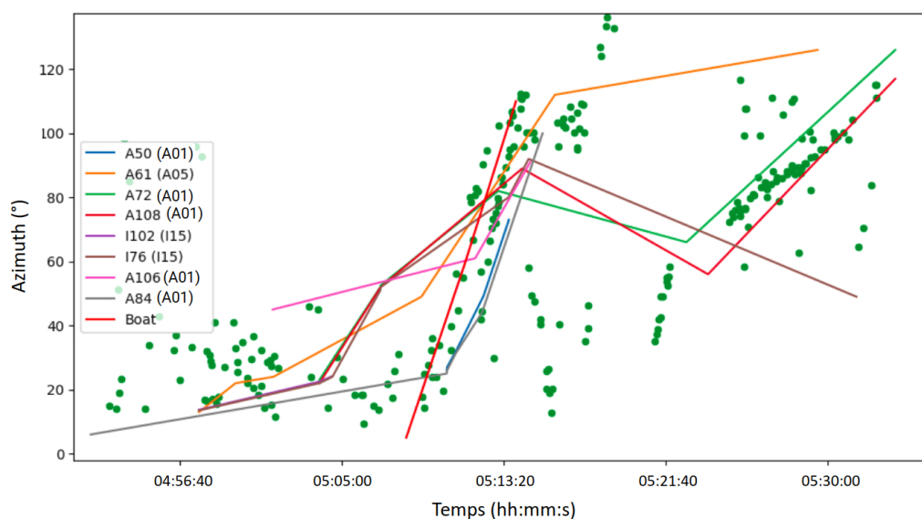
FIG. 4.33 – Graphique du passage du 11 août. Chaque point vert représente une vocalisation placée en azimut. Les différentes courbes sont les positions de chaque individu détecté visuellement.
