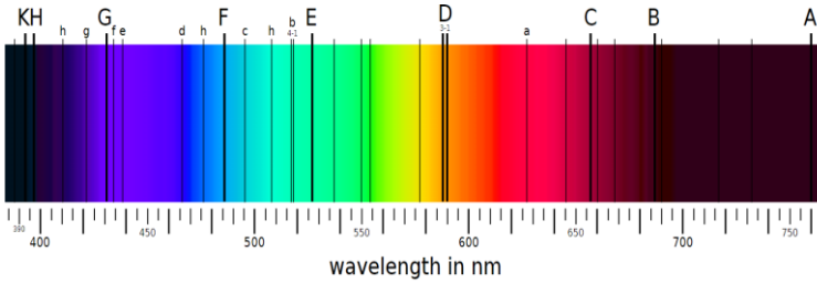
Fig. 5.3.f. Fraunhofer lines. Source: Gebruiker:MaureenV | Public Domain.
