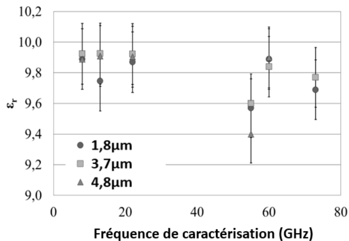
Figure II-30- Impact de la taille des grains sur la permittivité
