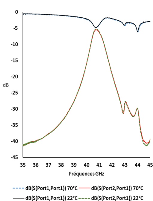
Figure IV-36- Mesure en température du filtre deux pôles TM-DAR 12%Ti entre 22°C et 70°C
