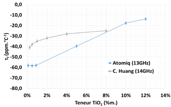
Figure II-46- Comparaison des facteurs de température des alumines dopées sans recuit à la littérature [53]
