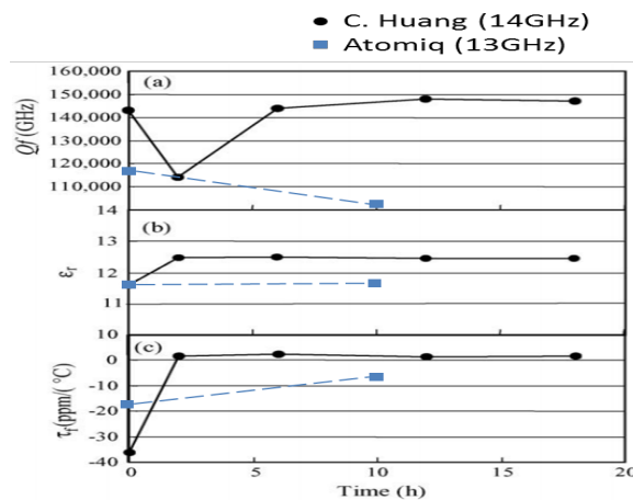
Figure II-47- Impact du temps de recuit à 1100°C sur \tau_f , \epsilon_r et Q^*f d'une céramique 0,9 \text{Al}_2\text{O}_3 – 0,1 \text{TiO}_2 [55]
