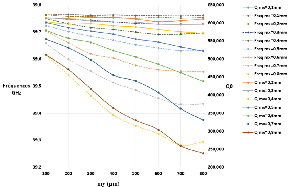
Figure IV-57- Variation du facteur de qualité et la fréquence (vers les basses fréquences) en fonction de la taille du motif
