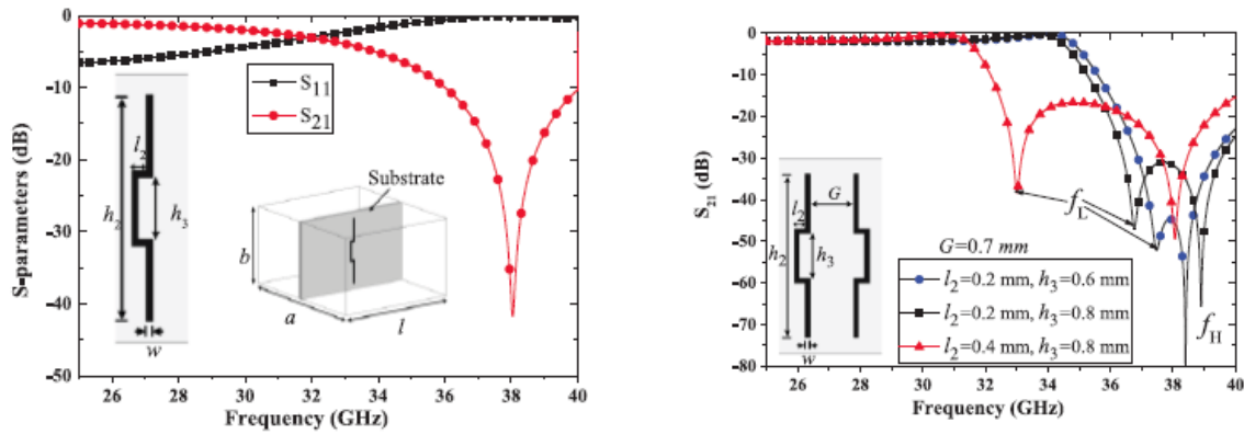
Figure I-30- Génération de deux zéros de transmission dans un guide d'onde à la fréquence haute [28] Enfin, il a assemblé toutes les parties pour réaliser la fonction de filtrage passe-bande. La Figure I-31 montre le filtre fabriqué ainsi que ses réponses fréquentielles simulée et mesurée. Deux zéros de transmission sont situés à 33,5 GHz et 36,6 GHz dans la bande d'arrêt supérieure et un troisième à 26 GHz dans la bande d'arrêt inférieure. Ces zéros améliorent grandement le niveau de rejection hors bande.
