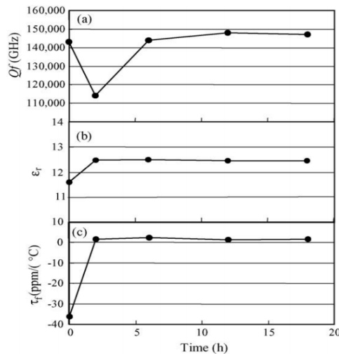
Figure II-10- Impact du temps de recuit à 1100°C sur \tau_f , \epsilon_r et (Q \cdot f) d'une céramique 90% Al 2 O 3 –10% TiO 2 frittée à 1350°C [56]
