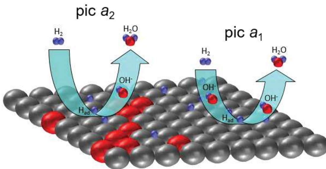
Fig. 3 Illustration schématique de la structure de l'électrode Ni activée in situ et un mécanisme d'activation HOR provisoire. Codes de couleurs: gris – \text{Ni}^0 , rouge – \text{NiO}_x .
