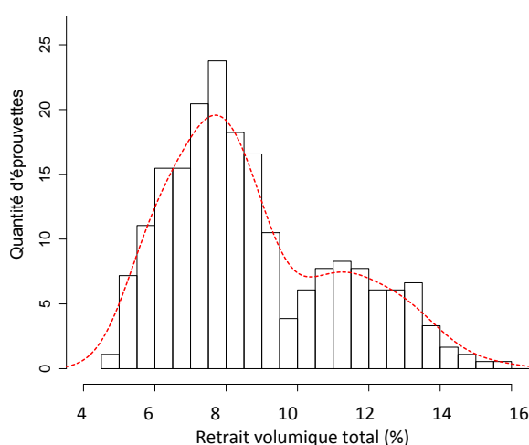
Figure 131 : Distribution des mesures de retrait volumique total pour tous les échantillons de B. guianensis .
