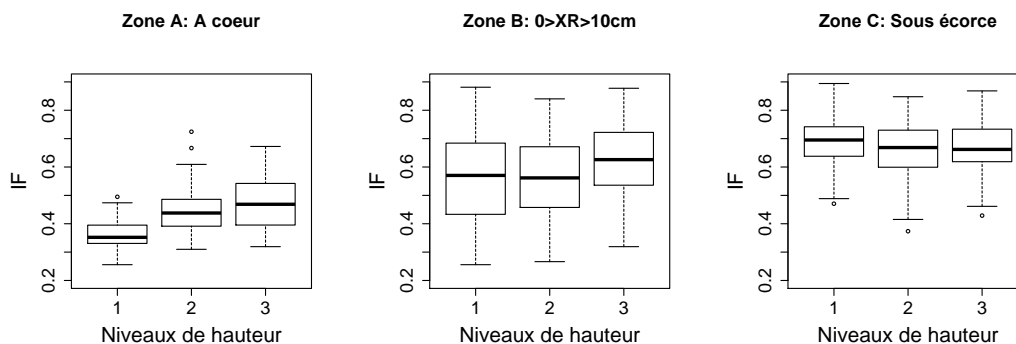
Figure 94 : Variabilité de l'infradensité à cœur, au centre et sous l'écorce selon le niveau de hauteur chez la bagasse. (Niveaux de hauteur : 1 : base ; 2 : mi-hauteur ; 3 : sous fourche).
