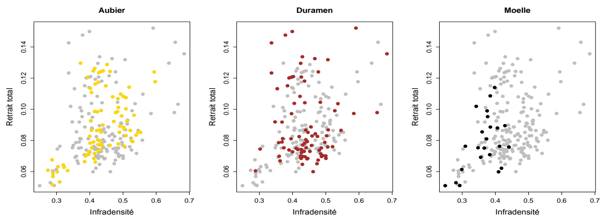
Figure 140 : Influence de l'infradensité sur le retrait volumique selon le type de bois chez C. alliodora . Les points gris permettent de situer les points d'aubier (en jaune), de duramen (en marron) et de moelle (en noir) en fonction du reste de l'échantillonnage. Aucun des trois sous-échantillonnages n'est corrélé à l'infradensité.
