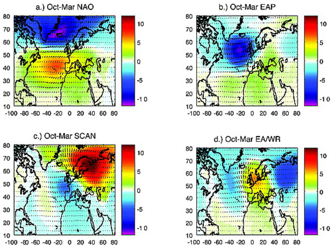
Fig. 1.2 Figure extraite de Josey et al. (2011) I.4. Champs composites des anomalies de pression de surface hivernale (octobre-mars) NCEP de 1958 à 2006 (en couleurs) et vent à 10m (vecteurs) pour les modes de variabilité suivants : (a) NAO, (b) EA, (c) SCAN, and (d) EA/WR. Le vecteur en bas à gauche de chaque cadre correspond à une vitesse de vent de 5 \text{ m s}^{-1} .
