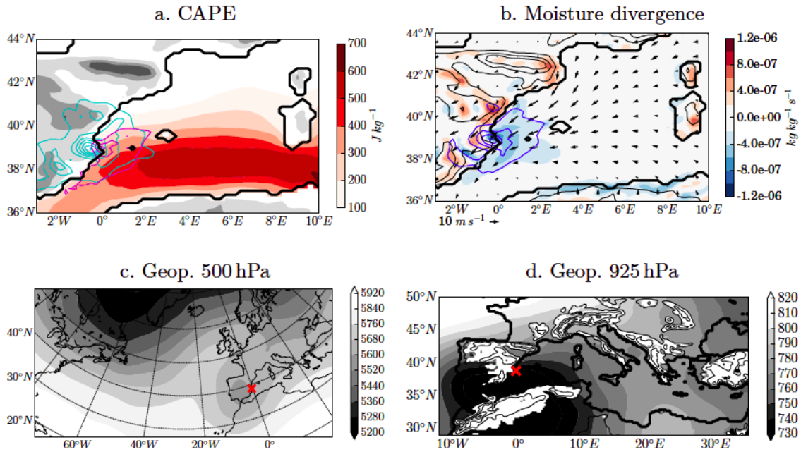
Fig. 6.3 Composite pour les événements présentant des différences négatives SST_{CPL} - SST_{SMO} . a : CAPE (couleurs, J kg^{-1} ), contours bleu clair : précipitations explicites, contours magenta : précipitations paramétrisées, contour tous les 10 mm. Nuances de gris : topographie, contour tous les 500 m. b : couleurs : divergence d'humidité ( kg kg^{-1} s^{-1} ), contours bleus : précipitations totales, contour tous les 20 mm, contour noir : topographie tous les 500 m. c : Hauteur de géopotential à 500 hPa à 1200 UTC (m). d : hauteur de géopotential à 925 hPa à 1200 UTC.
