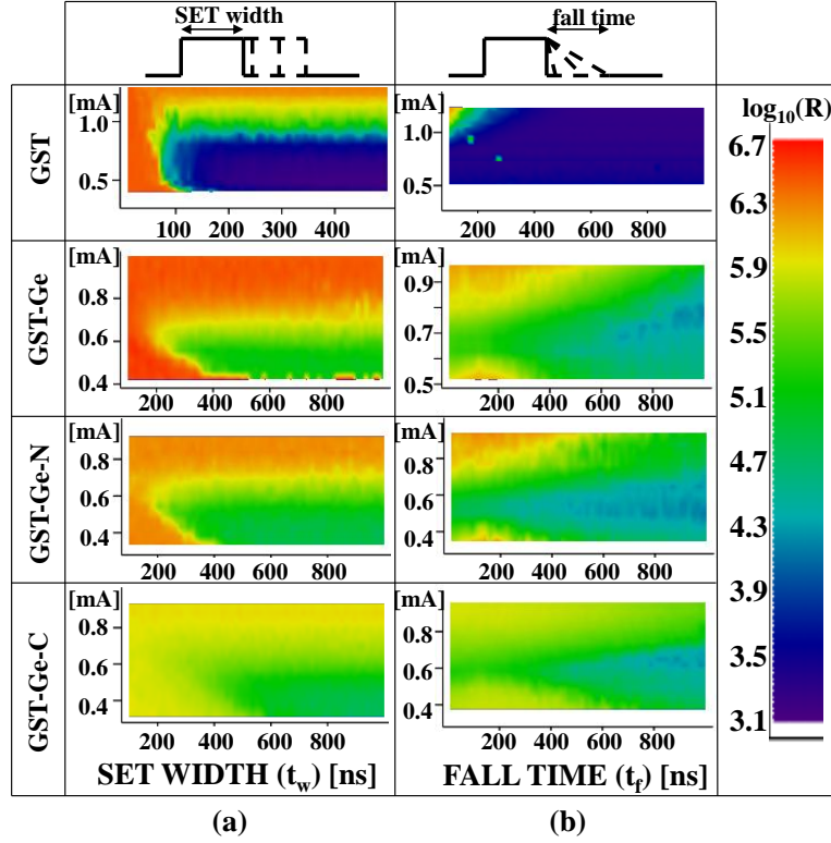
Figure 7: Cartographies de recristallisation du GST et des matériaux basés sur GST riche en Ge lorsque la durée (a) ou le temps de descente (b) de l'impulsion de SET augmentent.
