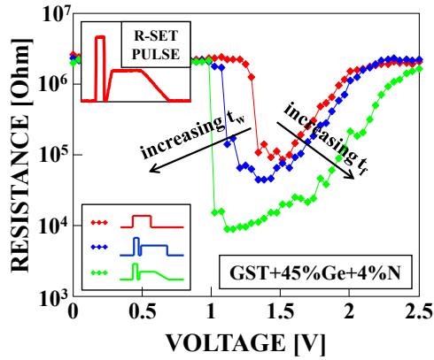
Figure 9: Effet de l'impulsion R-SET (en médaillon) sur les courbes de programmation pour GST+45%Ge+4%N.
