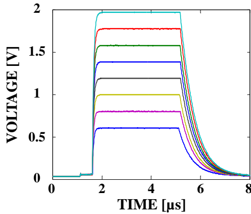
Figure 24: Impulsions de RESET d'amplitude variée mesurées.
