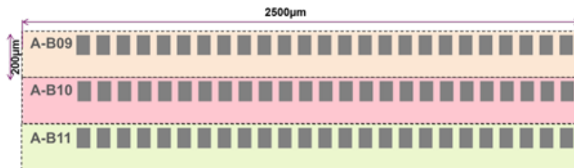
Figure 16: Lignes de scribe pour le générateur d'impulsions R-SET.
