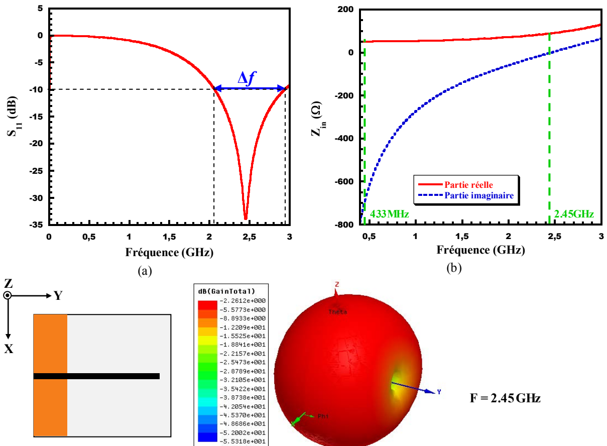
Figure. II.18: Résultats de simulation de l'antenne monopôle :(a) Module du coefficient de réflexion S_{11} , (b) Impédance d'entrée Z_{in} et (c) Diagramme de rayonnement 3D ( F=2.45\text{GHz} ).
