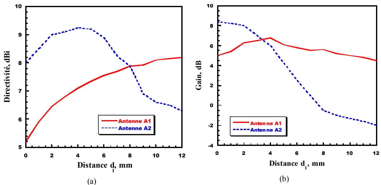
Figure III.18: Effet de la distance d_1 de couplage à la fréquence F_R , à la directivité simulée (a) et le gain (b) pour les configurations A1 ( F_R = 1.55 ) et A2 ( F_R = 1.75 ).
