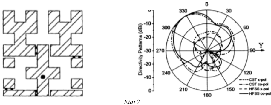
Figure I.25: Exemple d'antenne fractale reconfigurable en rayonnement.
