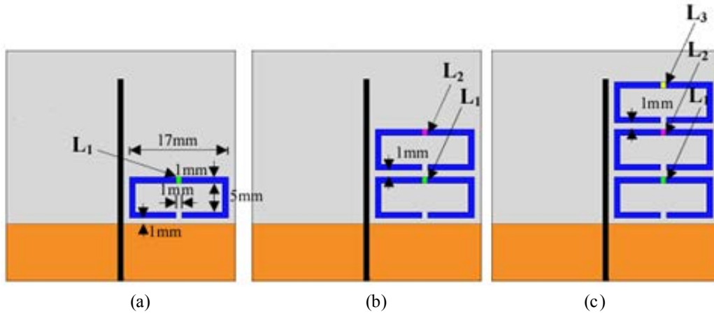
Figure II.26: Géométries et dimensions des antennes proposées : (a) Antenne A1; (b) Antenne A2 et (c) Antenne A3.
