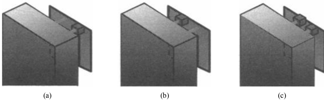
Figure 1.7 : Placement d'un fragment de matériau magnétique selon trois configurations : (a) insertion autour de l'alimentation et (b) insertion autour du court-circuit et (c) insertion autour de l'alimentation et du court-circuit.
