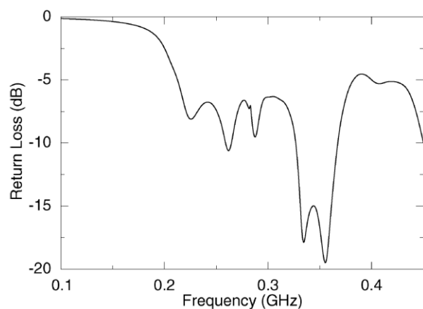
Figure 1.8: Exemple d'antenne à matériaux magnéto-diélectriques : (a) Antenne réalisée et (b) Coefficient de réflexion.
