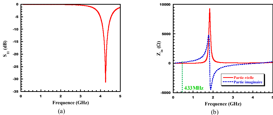
Figure II.21: Résultats de simulation de la boucle seule : (a) Module du coefficient de réflexion S_{11} , (b) Impédance d'entrée Z_{in} .
