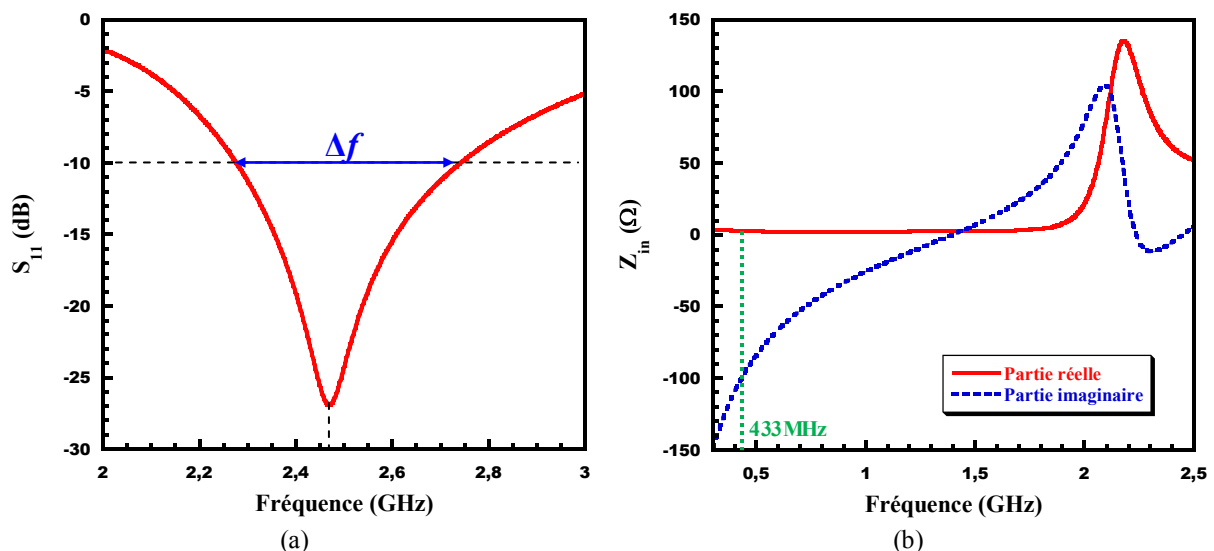
Figure. II.34: Résultats de simulation de l'antenne monopôle : (a) Module du coefficient de réflexion S_{11} (dB), (b) Impédance d'entrée Z_m ( \Omega ).
