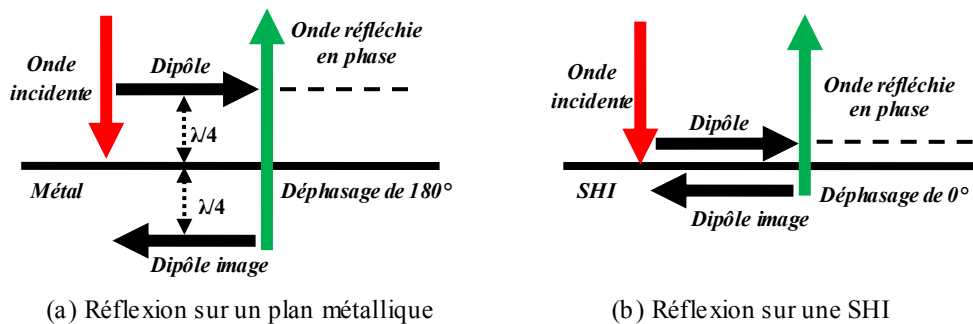
Figure I.14: Principe de l'augmentation de la directivité par réflexion.
