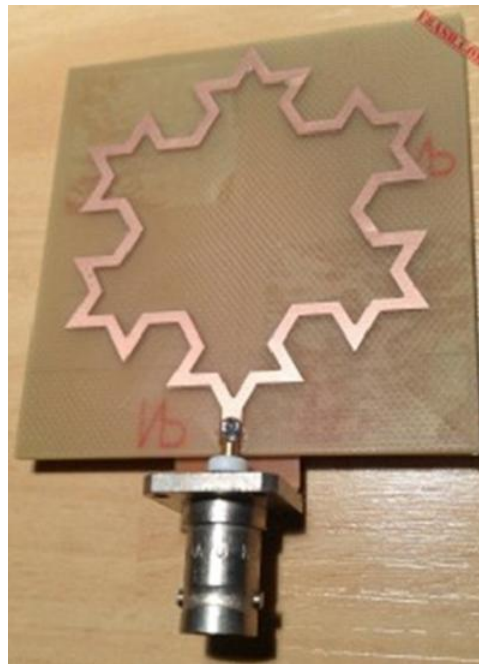
Figure I.4: Antenne imprimée à fractales de Koch d'ordre 3.
