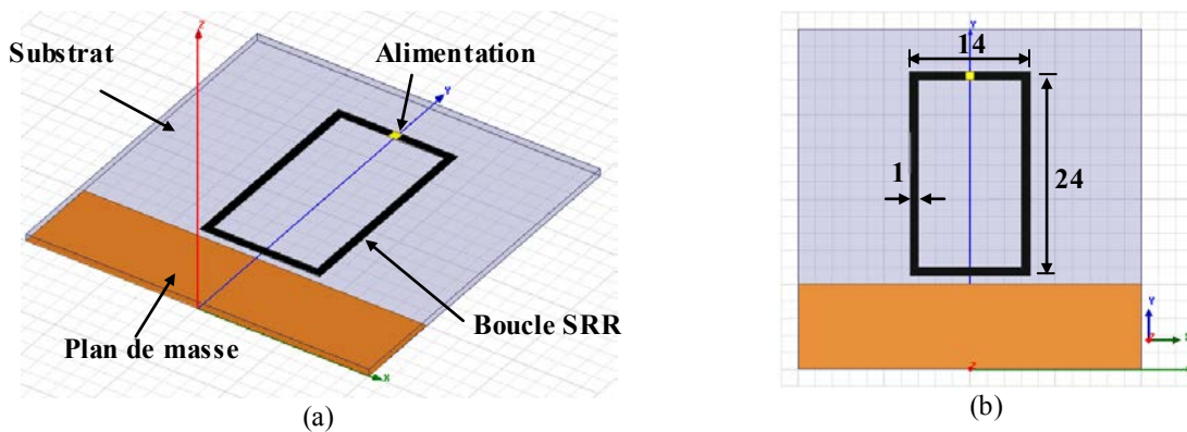
Figure II.20: Boucle seule : (a) Modèle HFSS, (b) dimensions (mm).
