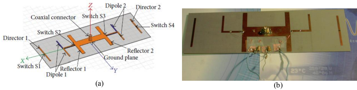
Figure 1.29: Antenne reconfigurable en diagramme par l'utilisation d'une ligne commutable : (a) Structure de l'antenne et (b) Photo du prototype.
