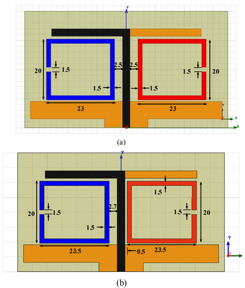
Figure II.42: Géométries et dimensions (mm) des antennes proposées: (a): Antenne A1 (b): Antenne A2.
