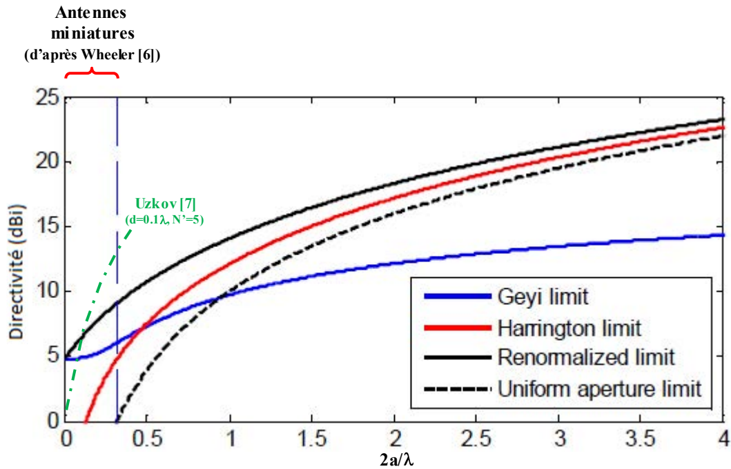
Figure III.1: La limite renormalisée proposé dans [III.5] comparés à la limite de Harrington et à la limite de Geyi. La directivité d'un réseau uniforme est rappelée à titre de comparaison. La ligne verticale discontinue définie la limite des antennes miniatures proposée dans [III.6]
