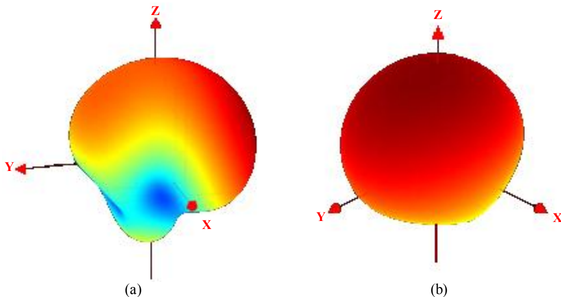
Figure IV.9: Diagrammes de rayonnement mesurés pour l'antenne à un élément SRR: (a) Etat A F= 1.59 GHz et (b) Etat B: F= 1.76 GHz.
