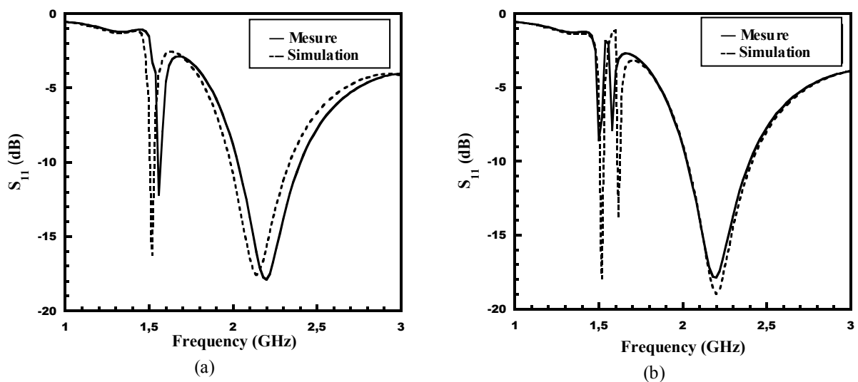
Figure II.47: Le coefficient de réflexion simulés et mesurés : (a) antenne A1 et (b) antenne A2.
