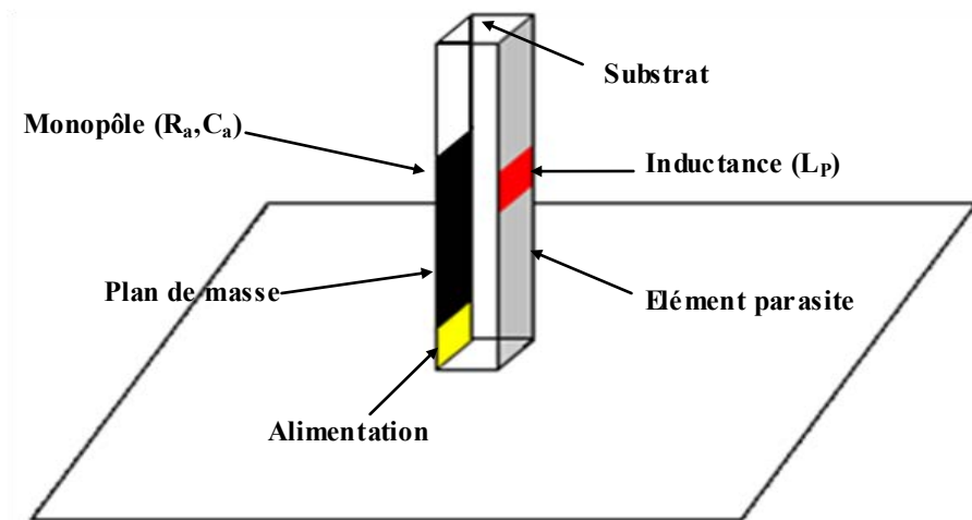
Figure II.7: Schéma de l'antenne avec un élément parasite intégrant une inductance.
