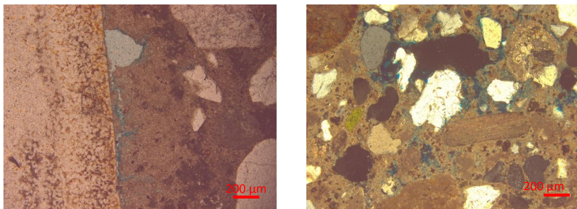
Figure 2-23. À gauche : GRIm, porosité en périphérie des grains ; à droite : GRIm porosité à l'interface pâte/granulat
