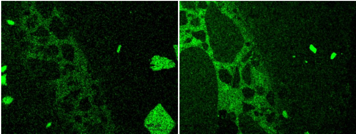
Figure 3-11. Microscopie électronique à balayage, cartographie élémentaire du K (potassium) au niveau de l'interface ancienne pâte / nouvelle pâte de (a) un granulat de BRL 0,6 ; (b) un granulat de BRI 0,6
