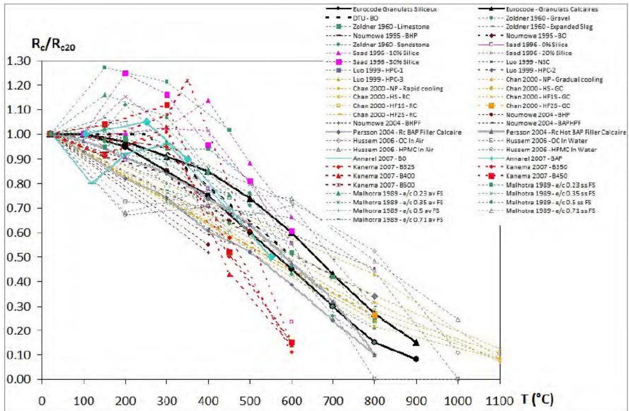
Figure 1-11. Résistances à la compression de bétons à chaud de bétons mesurée par différents auteurs [Fare 2009]
