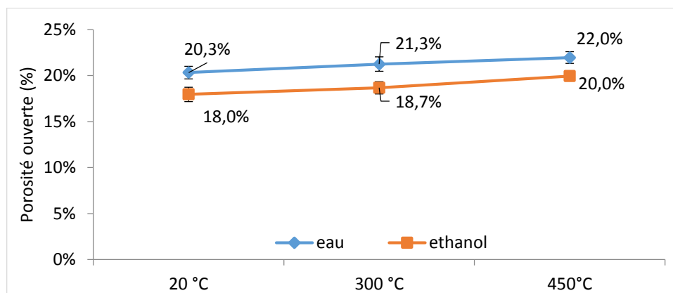
Figure 4-17. Comparaison de l'évolution de la porosité à l'eau et à l'éthanol en fonction de la température du BRL 0.6
