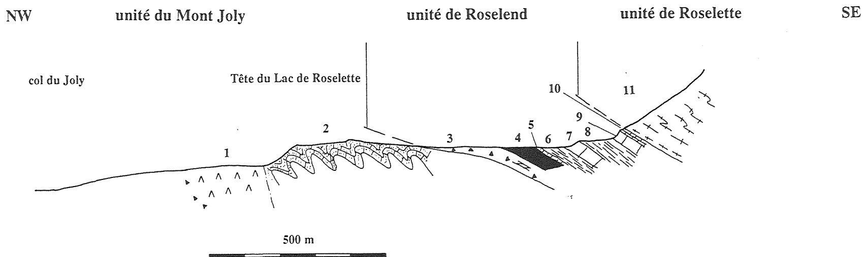
Fig. 48. Coupe de l'unité de Roselend des abords du col du Joly à l'Aiguille de Roselette (légende dans le texte).
