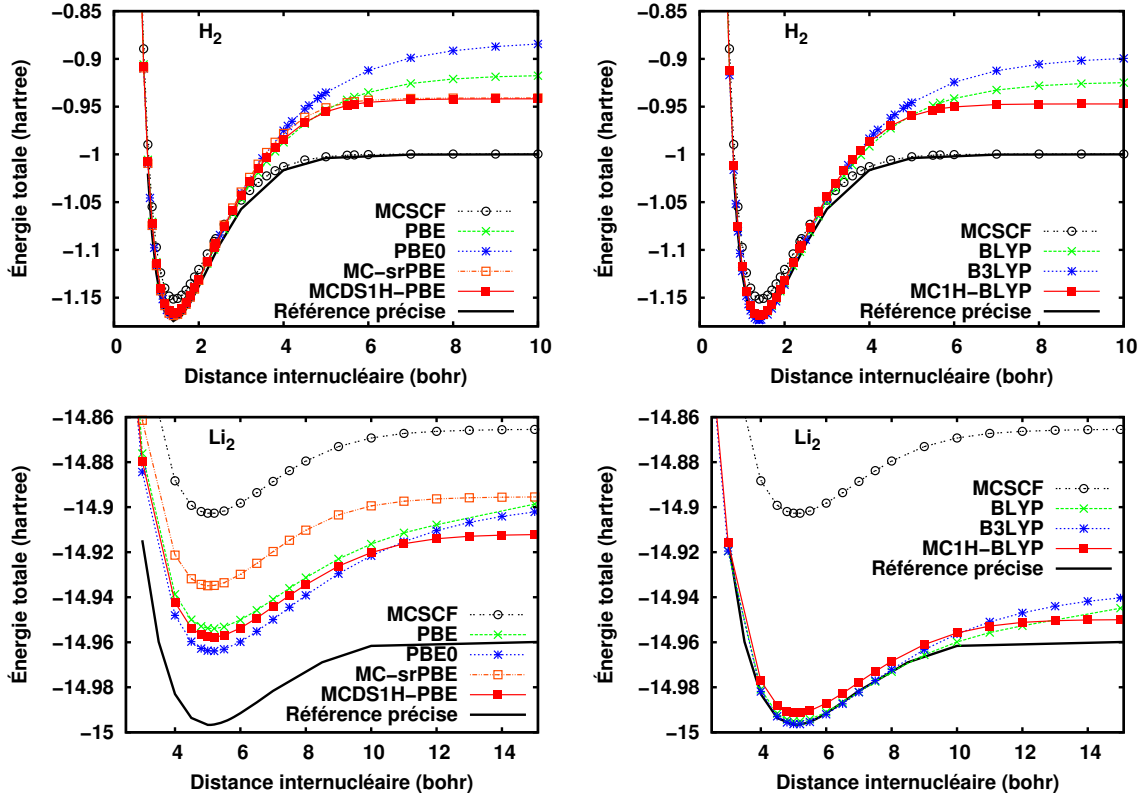
FIGURE 9: Courbes d'énergie potentielle de \text{H}_2 et \text{Li}_2 calculées par MCSCF et par plusieurs méthodes basées sur les fonctionnelles d'échange-corrélation PBE (à gauche) et BLYP (à droite). Pour les approximations hybrides multiconfigurationnelles MCDS1H et MC1H, la valeur du paramètre est \lambda = 0.25 . Pour l'approximation hybride multiconfigurationnelle à séparation de portée MC-srPBE, la valeur du paramètre de séparation est \mu = 0.40 \text{ bohr}^{-1} . Pour toutes les méthodes multiconfigurationnelles, une fonction d'onde CAS incluant tout les orbitales de valence est utilisée. La base est cc-pVTZ. Les courbes précises sont prises de [165]. Voir [JT35] pour plus de détails.
