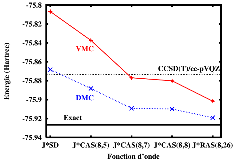
FIGURE 2: Amélioration systématique de l'énergie totale en VMC et en DMC pour la molécule C_2 pour une série de fonctions d'onde Jastrow-Slater à un seul déterminant (SD) et à plusieurs déterminants CAS(8,5), CAS(8,7), CAS(8,8) et RAS(8,26), avec la base Slater de Koga et al. [46]. Pour comparaison, l'énergie d'un calcul CCSD(T) avec la base cc-pVQZ est indiquée. Voir [JT14] pour plus de détails.
