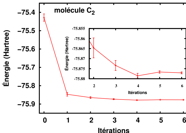
FIGURE 1: Convergence de l'énergie totale VMC pour la molécule C_2 lors de l'optimisation simultanée de 24 paramètres du facteur de Jastrow, 49 coefficients CSF et 64 paramètres orbitales pour une fonction d'onde Jastrow-Slater CAS(8,7) avec la base Slater de Koga et al. [46]. L'incertitude statistique sur l'énergie est initialement de 0.02 hartree et est diminuée par un facteur 2 à chaque itération jusqu'à 0.5 mhartree. L'insert est un élargissement des 5 dernières itérations. Voir [JT14] pour plus de détails.
