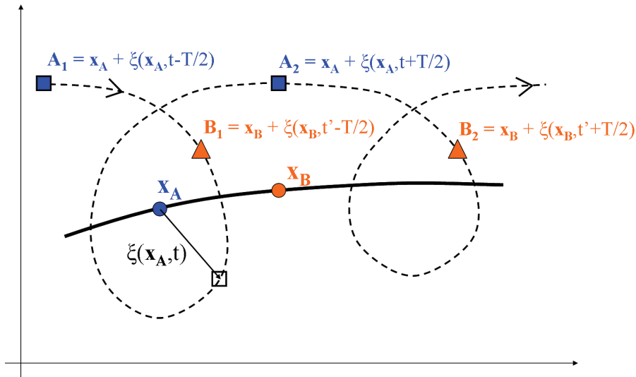
FIGURE II.1 – Schéma illustrant la définition du déplacement \xi(x, t) et de l'opérateur GLM. Le trait pointillé noir représente les positions instantanées d'une particule d'eau. Le trait plein noir représente les positions moyennes correspondantes. On signale à titre d'exemple deux positions moyennes particulières x_A et x_B ainsi que le vecteur \xi(x_A, t) à un instant t particulier. Les points A_1, A_2 et B_1, B_2 délimitent les portions de trajectoires dont la moyenne fournit les positions x_A et x_B respectivement.
