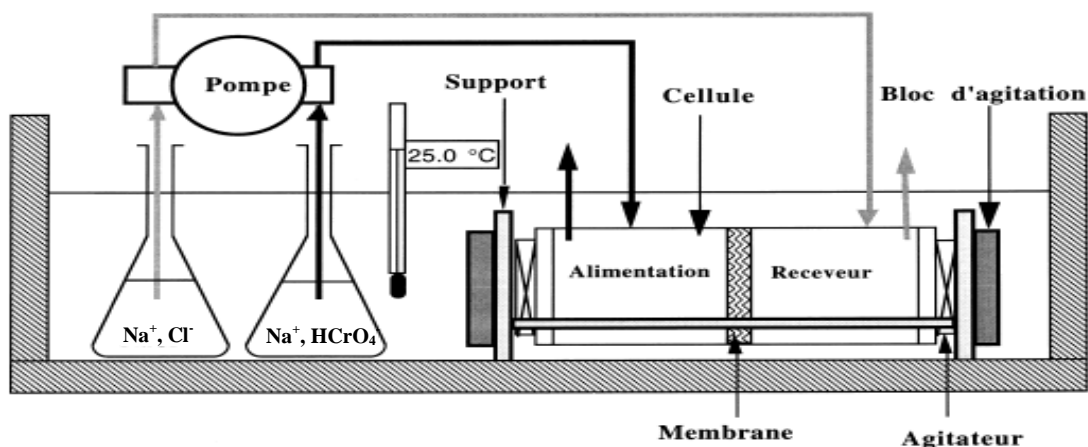
Figure IV- 3 : Montage expérimental.
