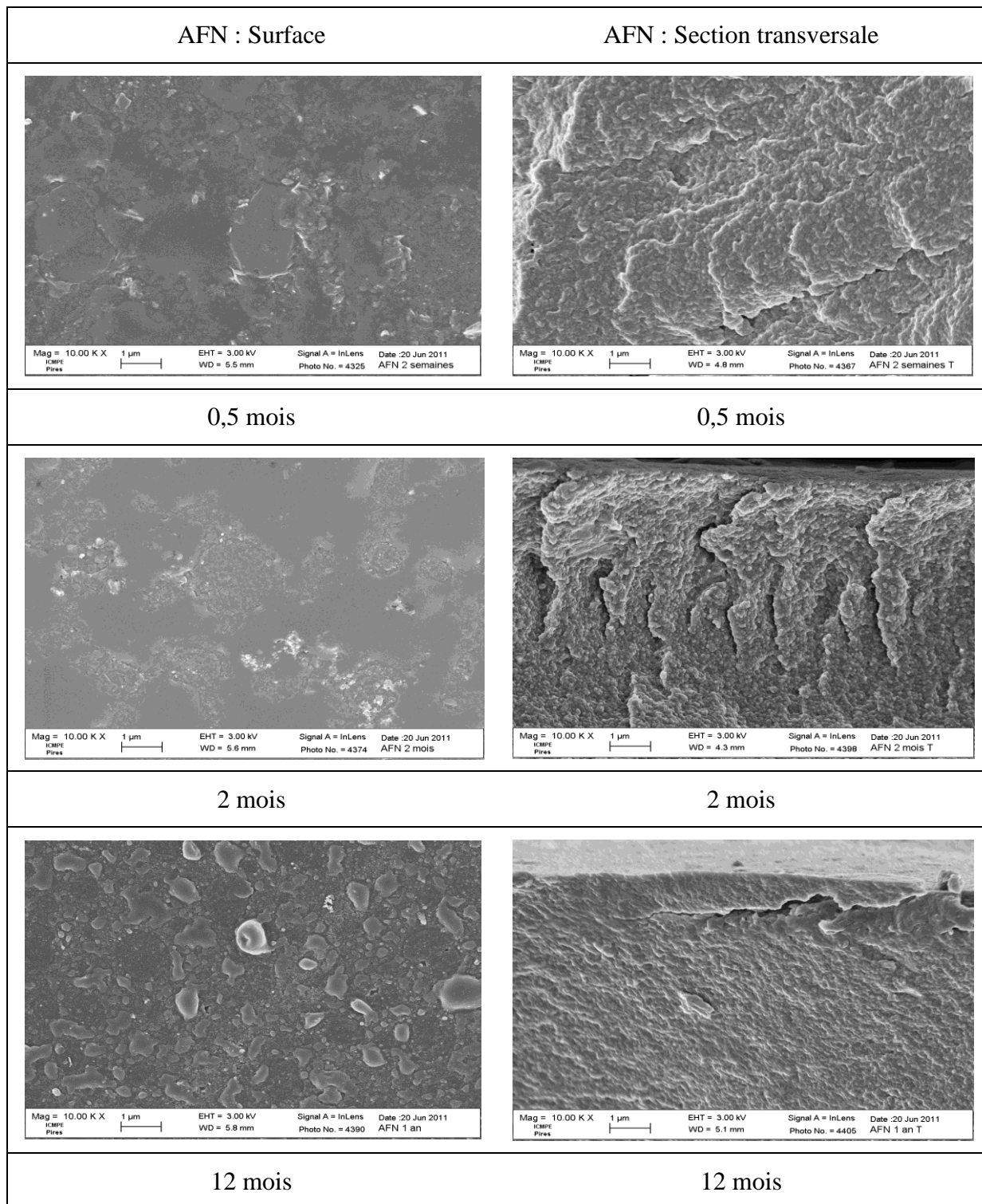
Figure IV- 22 : Clichés MEB de l'AFN (surface et section) pour différentes périodes d'immersion dans une solution 0,5 \text{ mol L}^{-1} en Cr (VI).
