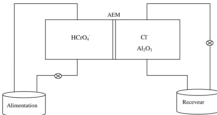
Figure IV- 25 : Schéma de fonctionnement du procédé obtenu par couplage de la DIC et de l'adsorption sur une alumine activée.
