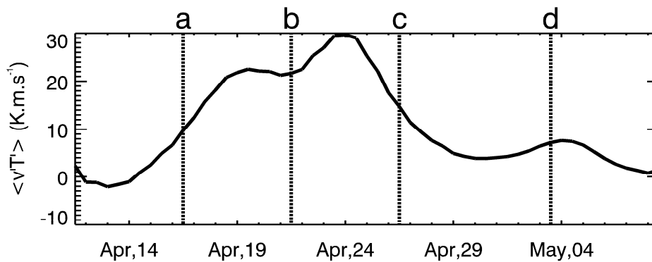
Figure 3.17. Évolution, entre 12 avril et le 9 mai 2007, du flux de chaleur \langle v'T' \rangle moyenné dans la bande de latitudes [45 ; 55]^\circ\text{N} à 30 hPa. Les barres verticales a,b,c et d indiquent les dates des cartes représentées figure 3.15.
