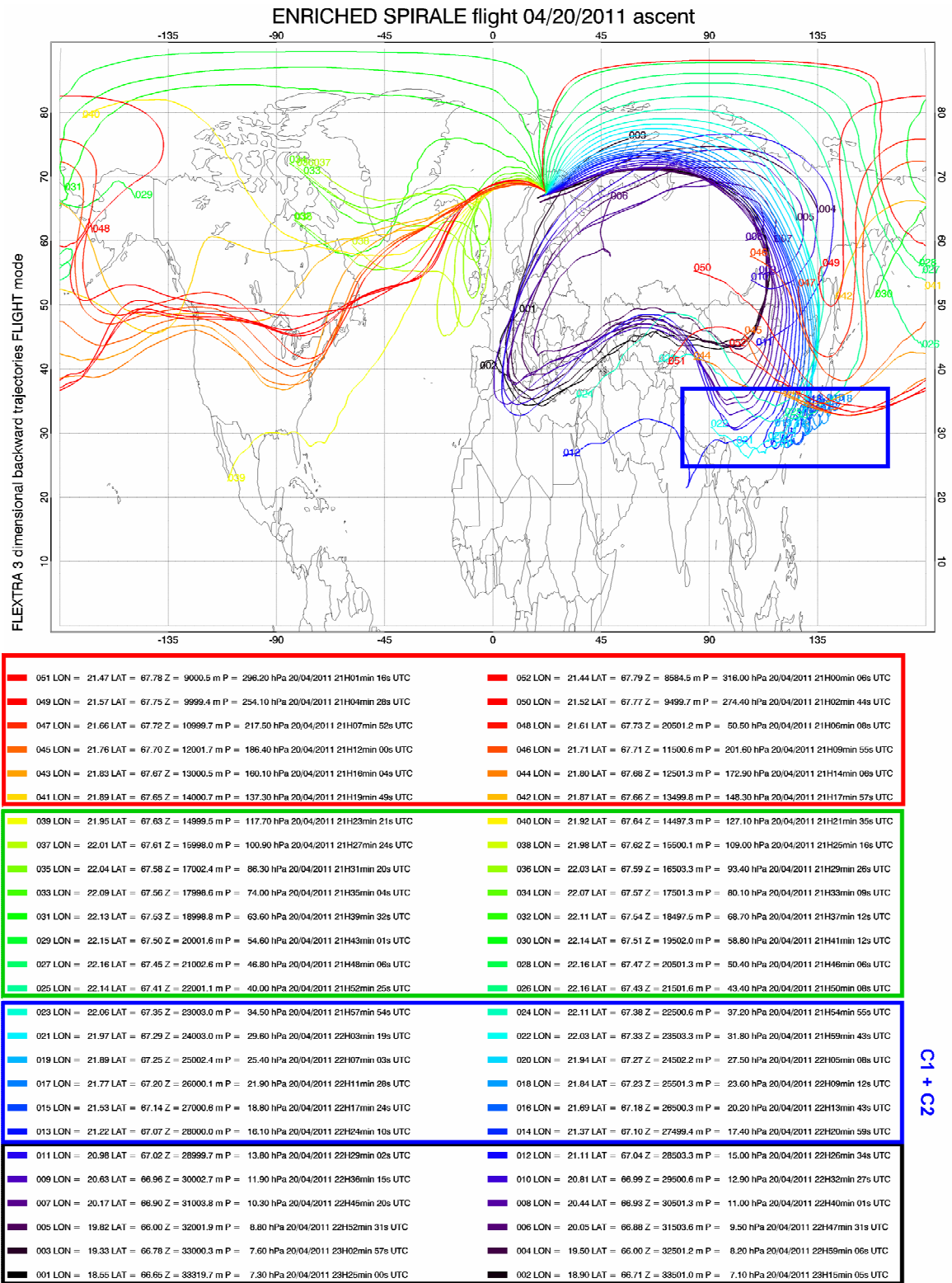
Figure 3.6. Rétro-trajectoires isentropes calculées à l'aide du modèle FLEXTRA [Stohl et al., 1995] le 20 avril 2011 au-dessus d'Esrange de 21h01 UT (à 9000 m) à 23h25 UT (à 33319 m). Chaque couleur est associées à une rétro-trajectoire.
