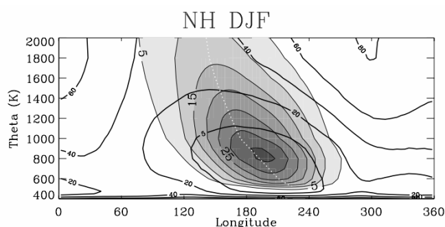
Figure 1.15. Coupe en longitude/altitude de la fréquence de présence climatologique (1991-2001) de l'anticyclone des Aléoutiennes (contours remplis) et du vortex polaire (contours). Les résultats sont donnés pour l'ensemble des mois de décembre, janvier et février. D'après Harvey et al. [2002].
