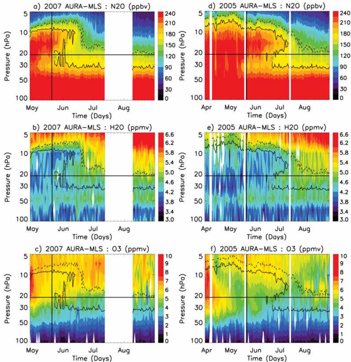
Figure 3.11. Évolution en fonction du temps et selon la pression (hPa) des rapports de mélanges de N_2O (en ppbv), H_2O (en ppmv) et O_3 (en ppmv) aux cœurs des FrIACs (cf figure 3.10) de 2007 (à gauche) et 2005 (à droite).
