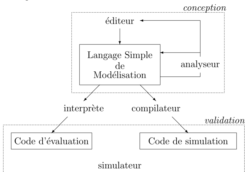
FIGURE 4.1 – Architecture de l'environnement
