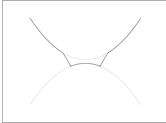
FIGURE 2.1 – saut entre deux composantes solutions
