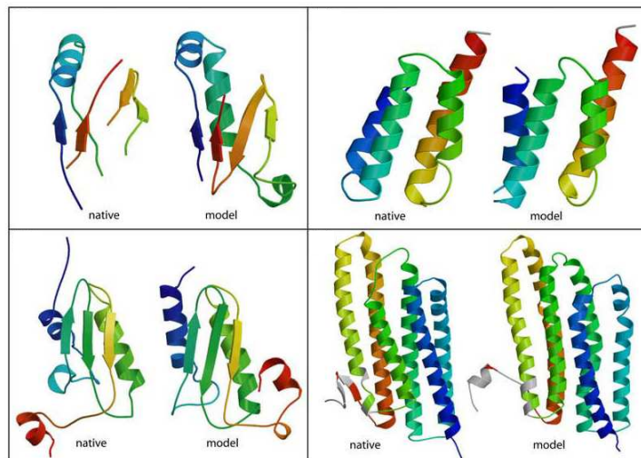
FIG. 1.6 – Prédiction de structures obtenues à l'aide du logiciel Rosetta [16] lors de la session CASP6 Image originale en couverture du journal PROTEINS : Structure, Function and Bioinformatics , volume 61 du 26 septembre 2005.
