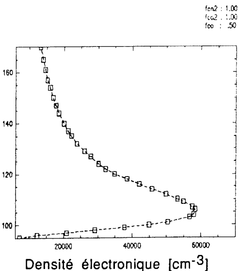
Figure 2-19 : Influence de changements de l'atmosphère neutre sur la densité électronique. Les facteurs f_{N_2} , f_{O_2} , et f_O écrits en haut à droite de chaque courbe sont les facteurs de division des densités de N_2 , O_2 , et O .
