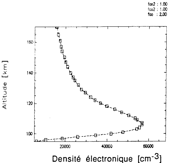
Figure 2-19 : Influence de changements de l'atmosphère neutre sur la densité électronique. Les facteurs f_{N_2} , f_{O_2} , et f_O écrits en haut à droite de chaque courbe sont les facteurs de division des densités de N_2 , O_2 , et O .
