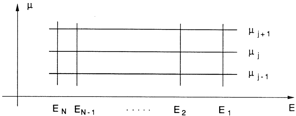
Figure 1-3: Pavés de grille en énergie et en angle.
