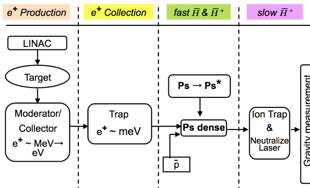
FIGURE 1.1 – Schéma de principe de l'expérience GBAR.
