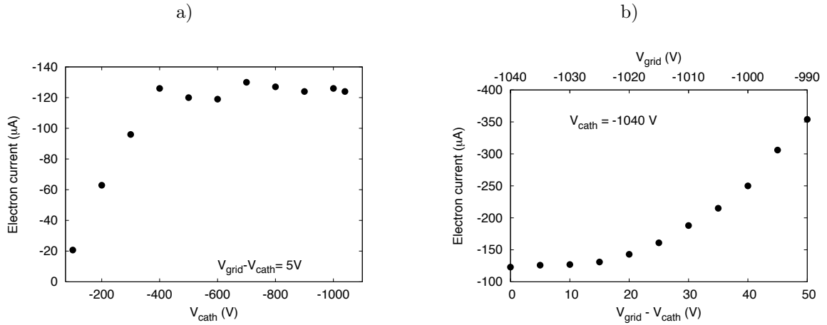
FIGURE 3.14 – Courant émis dans le piège avec toutes les électrodes à -50 V. a) Courant émis dans le piège en fonction du potentiel sur la cathode V_{cath} et V_{grid} - V_{cath} = 5 V. b) Courant émis dans le piège en fonction de la différence de potentiel V_{grid} - V_{cath} et V_{cath} = -1040 V.
