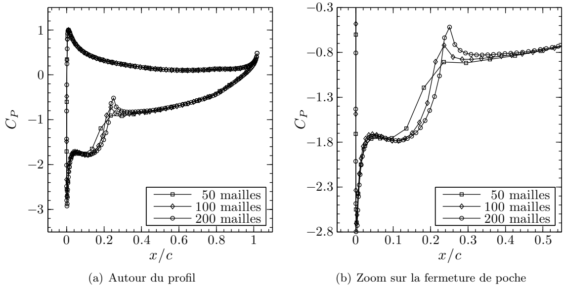
Figure 3.17. Effet du nombre de mailles sur la distribution des coefficients de pression ; profil NACA66(mod)-312 a=0.8 , \alpha = 6^\circ , milieu infini non-visqueux, \sigma_V = 1.75
