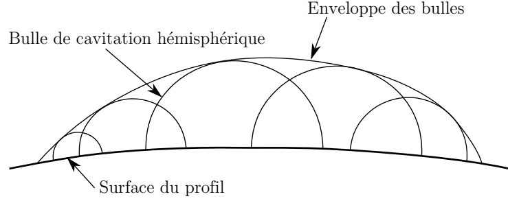
Figure 3.2. Schéma de la modélisation de la poche de cavitation à partir de l'enveloppe des bulles de cavitation
