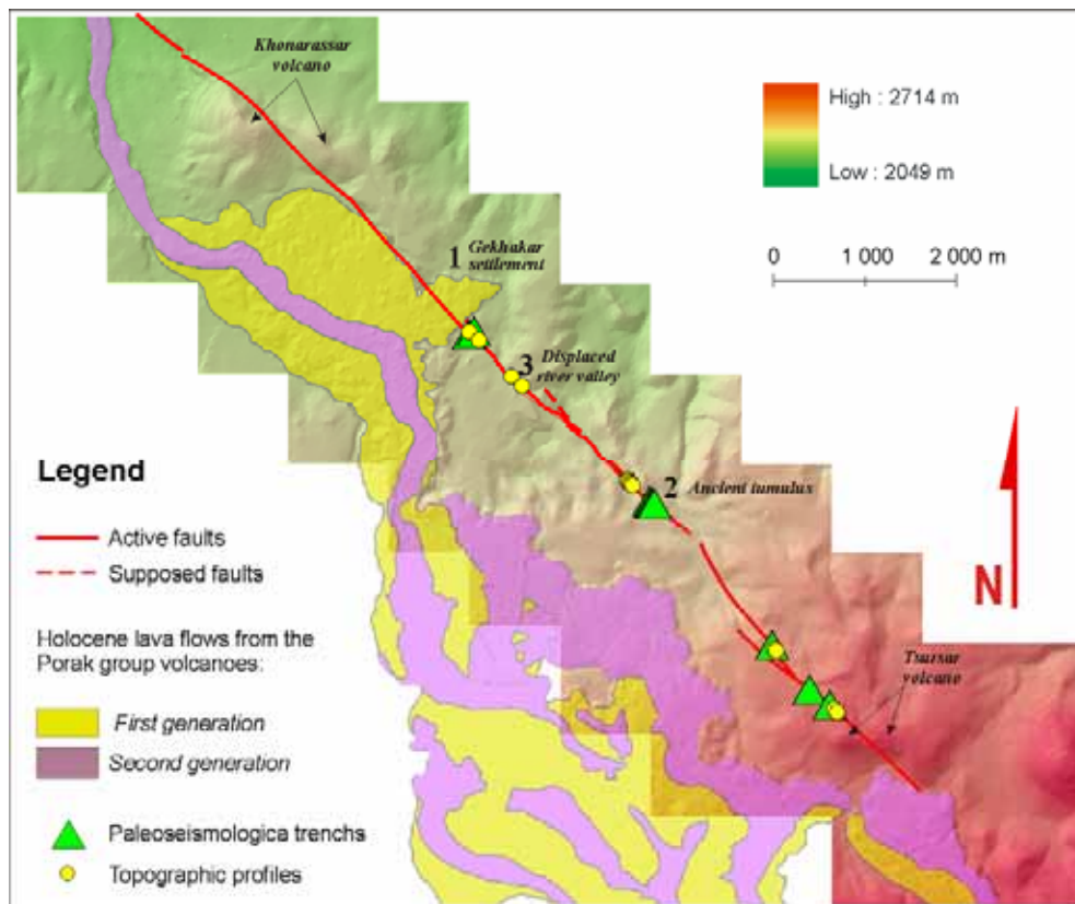
Figure III - 2 : Zones de recherches – A: la partie de Khonarassar-Porak du segment d'Artanish-Tskhuk de la faille PSSF de Pambak-Sevan-Suyunik (PSSF).
