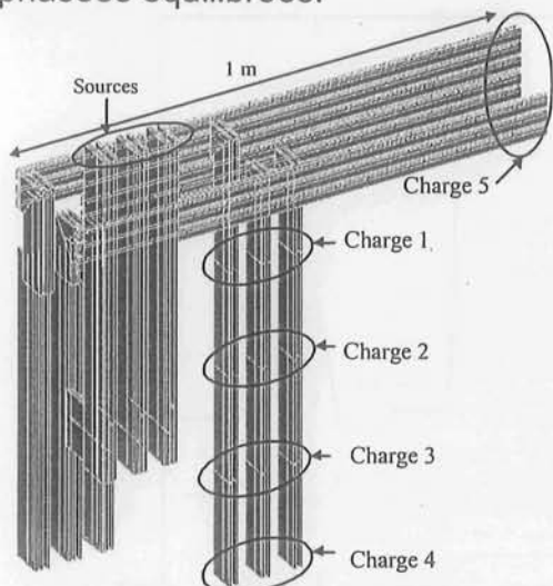
Fig. 39 : Jeux de barre Magellan « A »
