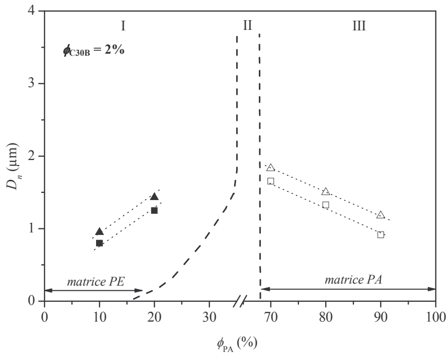
Figure 4.3.b. D_n en fonction de la fraction de PA à \phi_{C30B} = 2\% pour les deux modes d'élaboration : ( \blacktriangle, \triangle ) PE/PA/C30B – malaxage simultané. ( \blacksquare, \square ) PE/S 1 – malaxage à partir du mélange maître.
