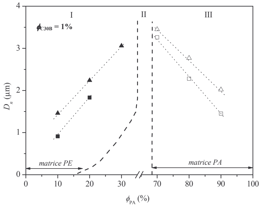
Figure 4.3.a. D_n en fonction de la fraction de PA à \phi_{C30B} = 1\% pour les deux modes d'élaboration : ( \blacktriangle, \triangle ) PE/PA/C30B – malaxage simultané. ( \blacksquare, \square ) PE/S 1 – malaxage à partir du mélange maître.
