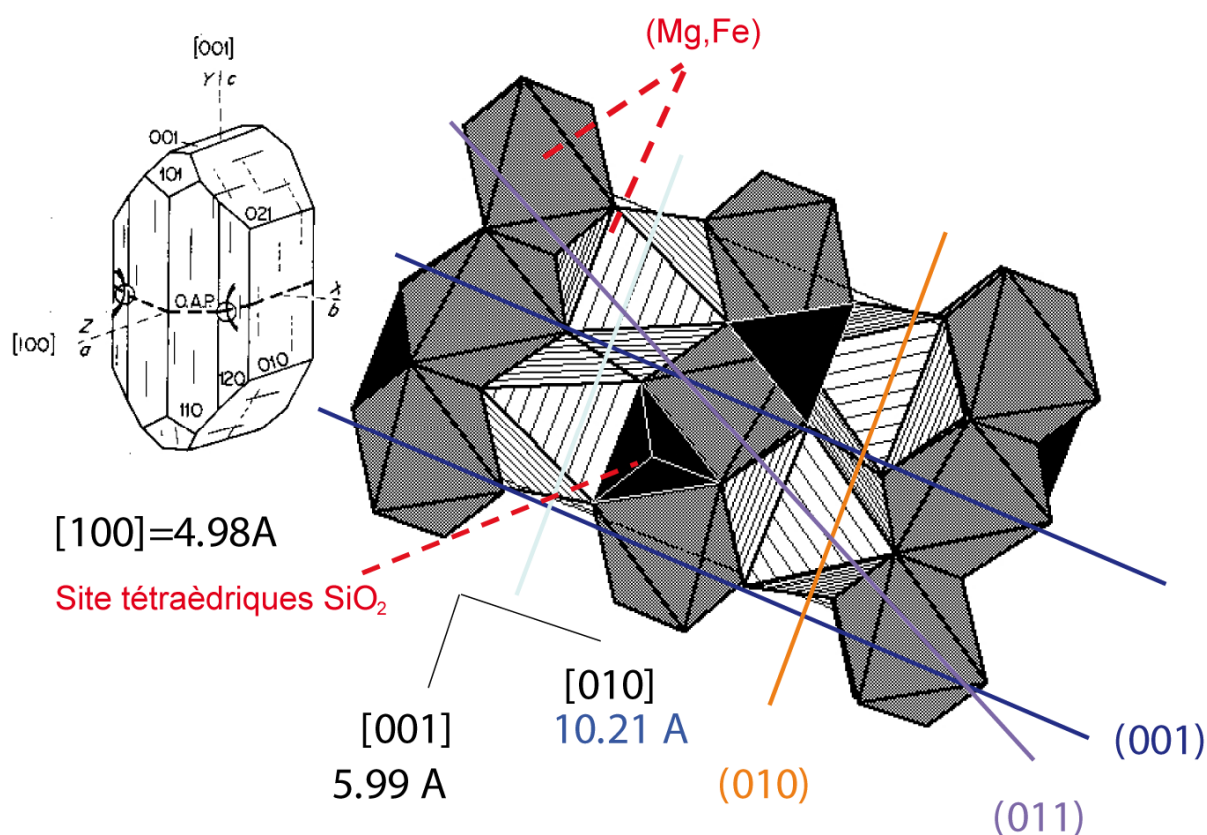
Figure 2-4: Représentation des systèmes des plans et direction de glissement dans le monocristal d'olivine
