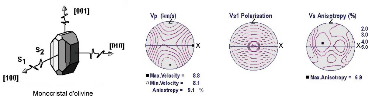
Figure 2-5: Données d'anisotropie sismique du monocristal d'olivine
