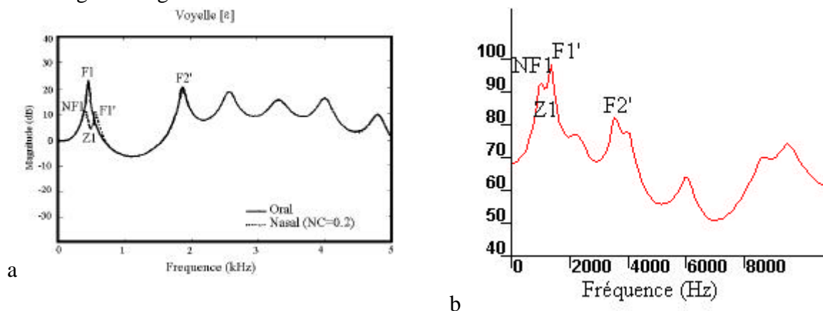
Figure 13: a : Identification des formants oraux (Fn), nasals (NFn) et des anti-formants nasals (Zn) après modélisation de la voyelle [ɛ], (Maeda, 2000), b : spectre acoustique de la voyelle [ɛ], calculé au milieu de la voyelle (loc1).
