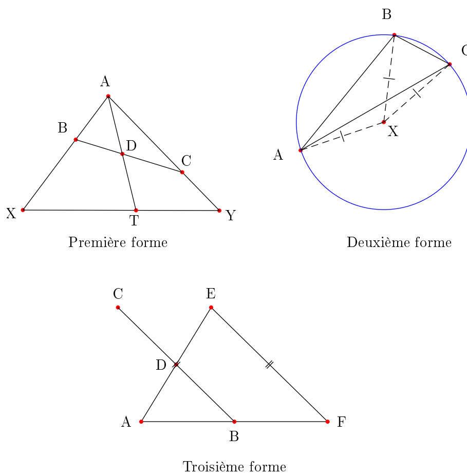
FIG. 2.4 – Axiomes d'Euclide
