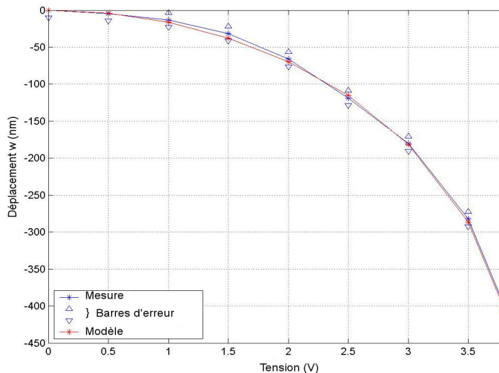
Figure 5-18 Courbe d'actionnement
