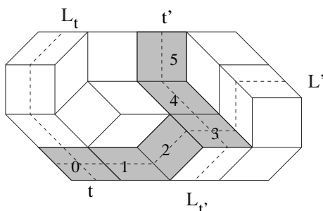
FIG. 3.20 – Le cas général, et les valeurs associées à un chemin de t à t' .
