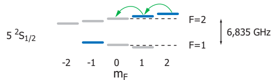
Abbildung 4.2: Energiediagramm des Grundzustandes 5^2s_{1/2} im Magnetfeld. Hervorgehoben sind die magnetisch gefangenen Zustände F = 2, m_F = 2 und m_F = 1 , und F = 1, m_F = -1 .
