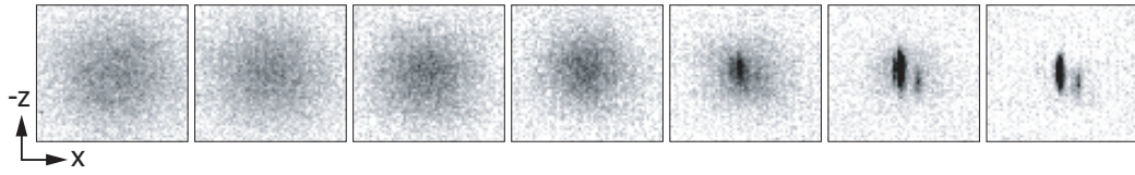
Abbildung 4.11: Von links nach rechts liegt der Endpunkt der letzten RF-Rampe um 10 kHz tiefer als im vorherigen Bild. Etwa im mittleren Bild tritt im Zentrum der isotropen, relativ verdünnten Wolke thermischer Atome ein dichter, anisotroper Kern hervor: das Bose-Einstein-Kondensat. Der kleine, rechts unterhalb des Zentrums liegende zweite dichte Kern ist ein Artefakt: Es handelt sich um Atome, die vermutlich beim Ausschalten der Falle in den magnetischen Unterzustand m_F = 1 transferiert und während der Expansion durch einen leichten Magnetfeldgradienten vom Hauptkondensat separiert wurden.
