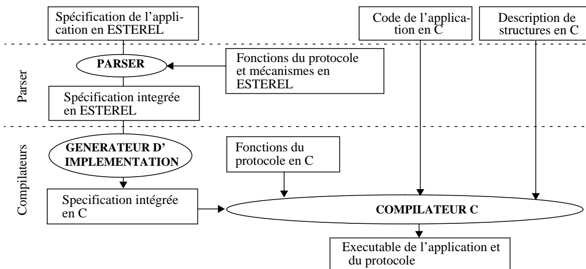
Figure 4: Architecture du compilateur de protocoles.
