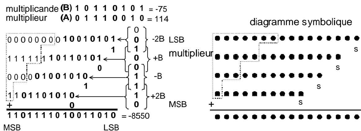
Figure 4.7. Une multiplication signée 8x8 de Booth2
