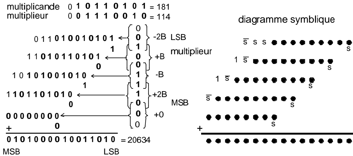
Figure 4.8. Une multiplication non signée 8x8 de Booth2
