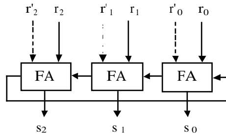
Figure 2.2. Un additionneur modulo 7 de deux résidus modulo 7
