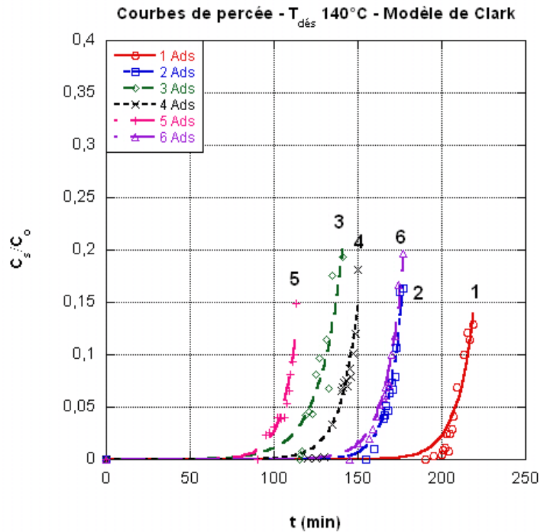
Figure III- 9 Courbes de percées successives à 25^{\circ}C alternées par des régénérations à 140^{\circ}C
