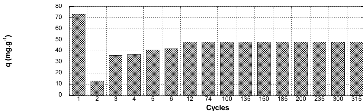
Figure IV- 11 Capacité de traitement en cycle
