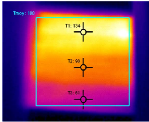
Figure III- 17 Thermogrammes de pièces de tissu FM 30 K contacts électriques \perp aux lisères
