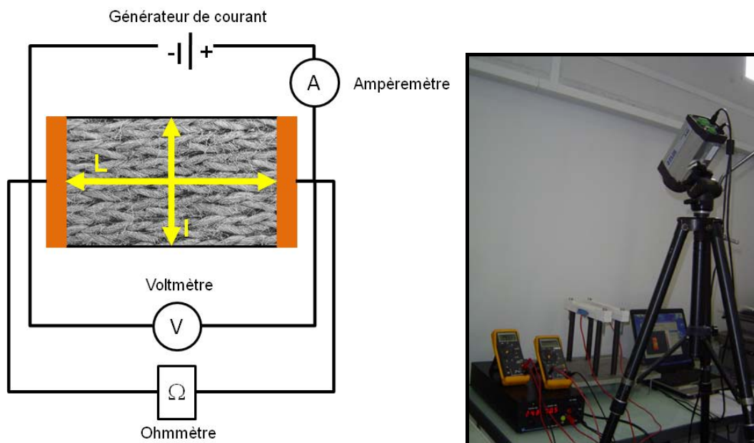
Figure III- 13 Principe général des caractérisations électriques
