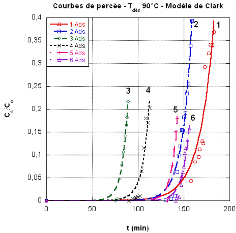
Figure III- 8 Courbes successives de percée à 25^{\circ}C alternées par des régénérations à 90^{\circ}C
