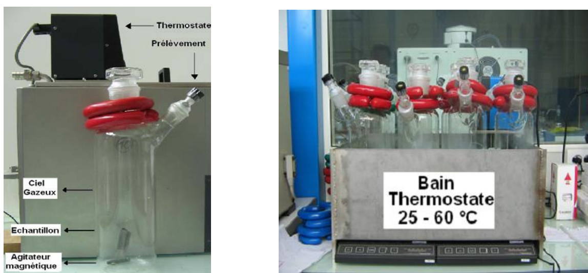
Figure II- 5 Montage expérimental pour l'adsorption en réacteur statique
