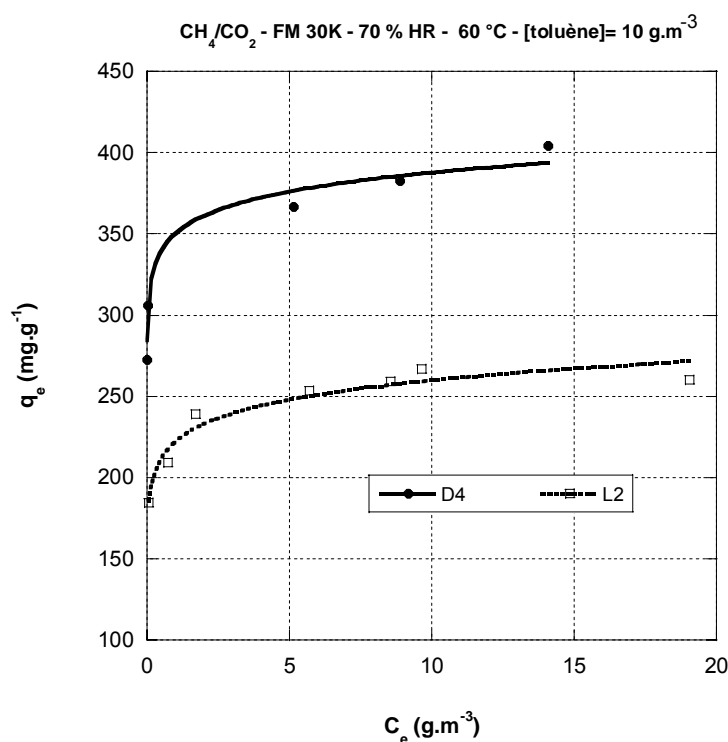
Figure II- 24 Isothermes d'adsorption du FM 30 K vis-à-vis du L2 et du D4 ( \text{CH}_4/\text{CO}_2 HR = 70% T = 60 \text{ }^\circ\text{C} , [toluène] = 10 \text{ g.m}^{-3} )
