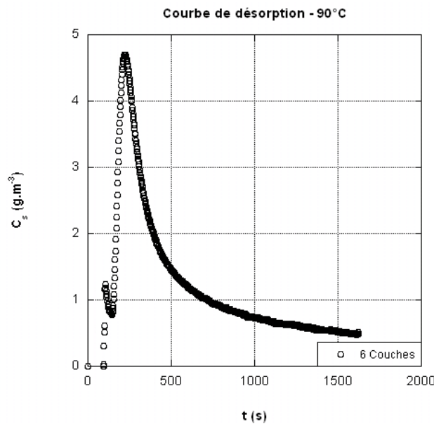
Figure III- 4 Profil de concentration du désorbat durant une régénération à 90°C
