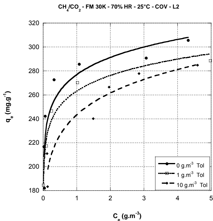
Figure II- 21 Isothermes d’adsorption du FM 30 K vis-à-vis du L2 en présence de toluène (CH 4 /CO 2 HR = 70% T = 25 °C)
