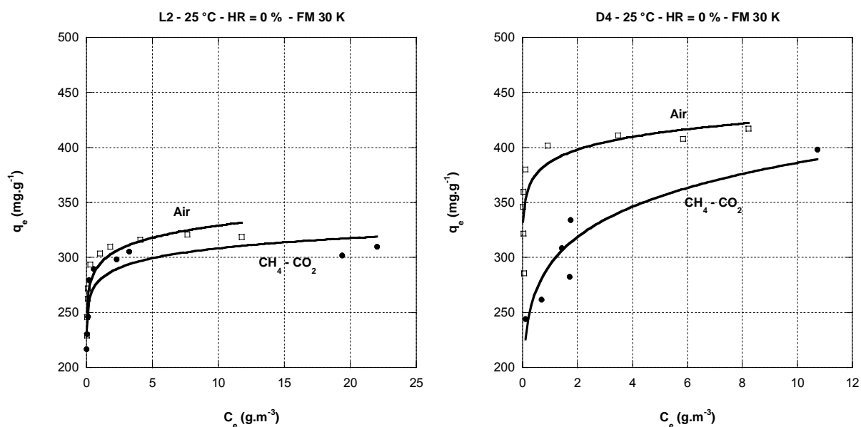
Figure II- 18 Isothermes d'adsorption sous air sec et en mélange CH 4 /CO 2 vis-à-vis du L2 et du D4
