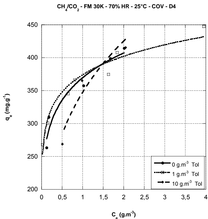
Figure II- 22 Isothermes d’adsorption du FM 30 K vis-à-vis du D4 en présence de toluène (CH 4 /CO 2 HR = 70% T = 25 °C)
