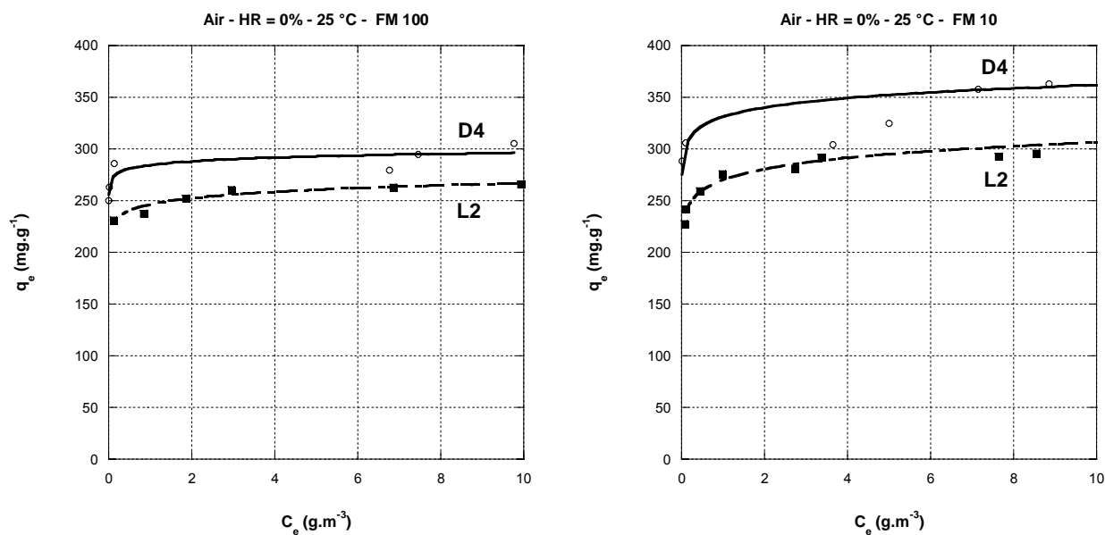
Figure II- 13 Capacités d'adsorption du L2 et du D4 sur des tissus de carbone activé
