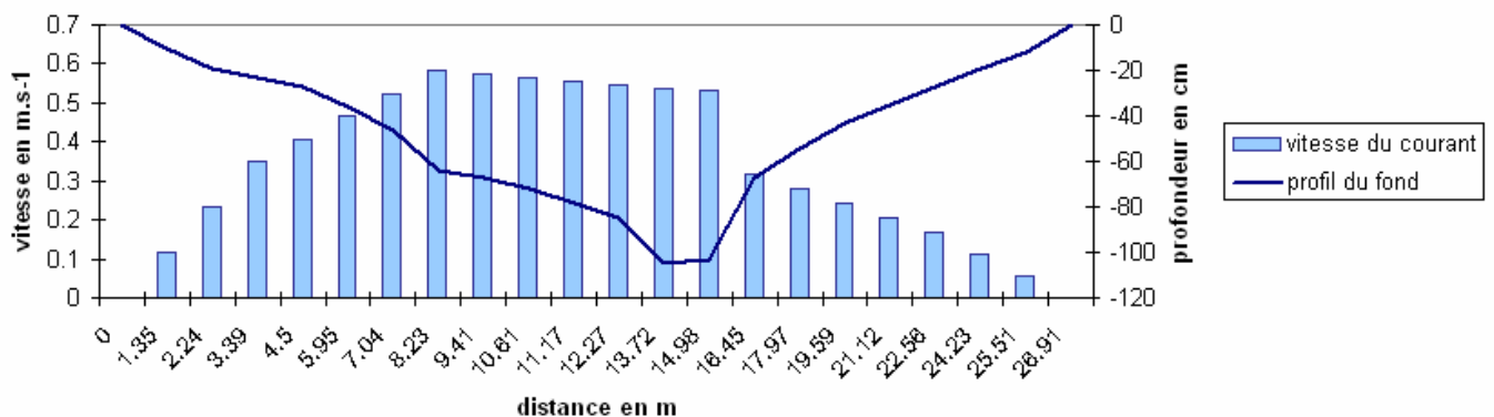
Figure 1 : Estimation du débit d'étiage dans les gorges près du point B10.
