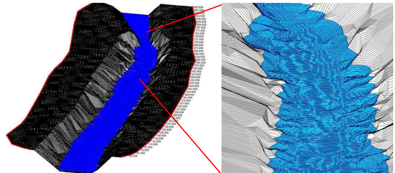
Figure 20 : Modélisation d'écoulement dans les gorges de la Bakeya obtenues avec le logiciel Hec-Ras.
