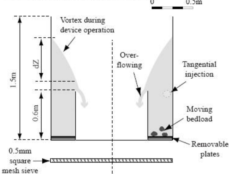
Figure 1 : Les dispositifs expérimentaux de simulation de l'érosion d'après Attal [2003].
