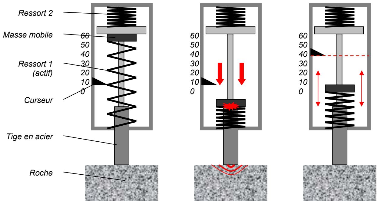
Figure 28 : Schémas fonctionnels d'un marteau de Schmidt.
