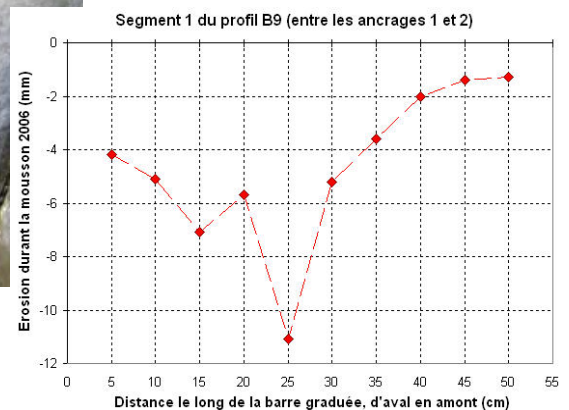
Figure 9 : Augmentation de l'érosion au voisinage des fissures, exemple du profil B9, segment 1 (base).
