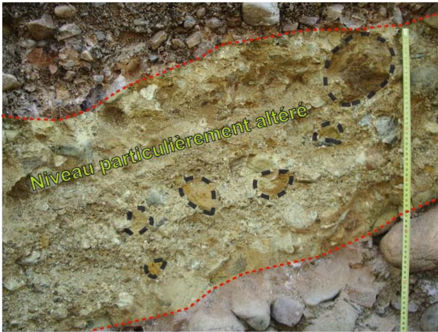
Figure 23 : Altération des galets dans les conglomérats Siwaliks Sup.
