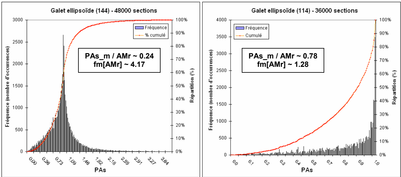
Figure 14 : Répartition des PAs pour un galet oblate (144) et un galet prolate (114). La répartition pour un galet prolate ressemble à celle d'une sphère. Le facteur correcteur est calculé pour plus d'un million de sections. Plus le galet est oblate, plus la correction à appliquer est importante.
