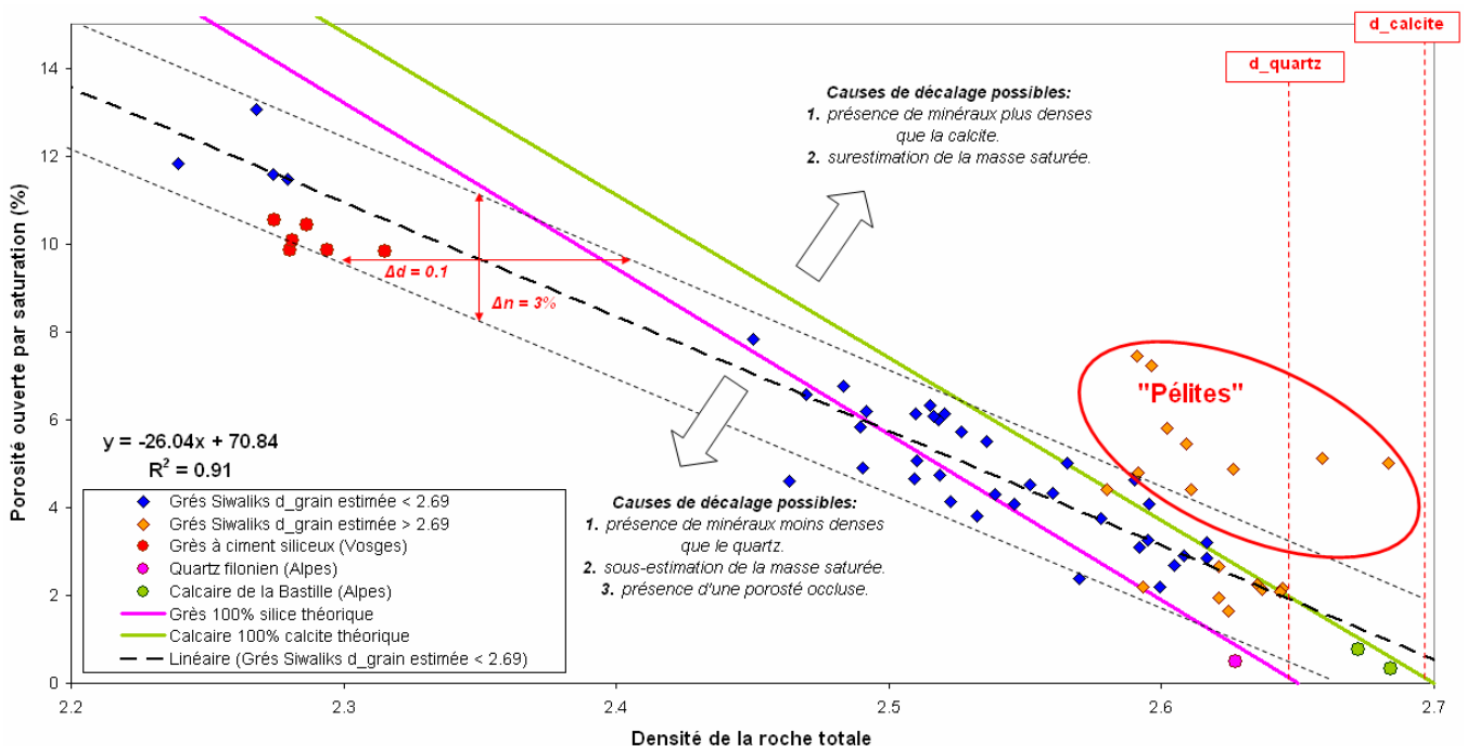
Figure 7 : Corrélation entre la densité de la roche et la porosité ouverte par saturation.
