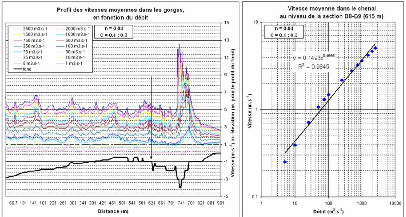
Figure 22 : Vitesse du courant dans les gorges, effet des variations de débit.
