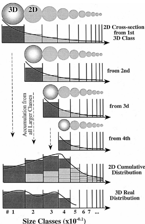
Figure 25 : Schématisation de l'effet de coupe, différence entre le spectre granulométrique 2D et le spectre granulométrique 3D, cas de sphères [Sahagian and Prousevitch, 1998].
