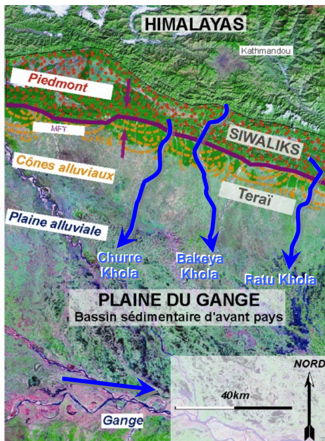
Figure 2 : Localisation du laboratoire naturel : les rivières des Siwaliks du Népal Central.
