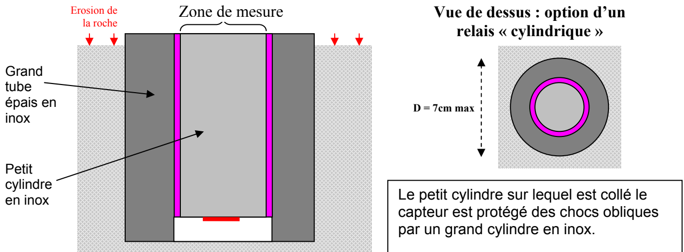
Figure 18 : Erosion différentielle et protection du cylindre en métal.
