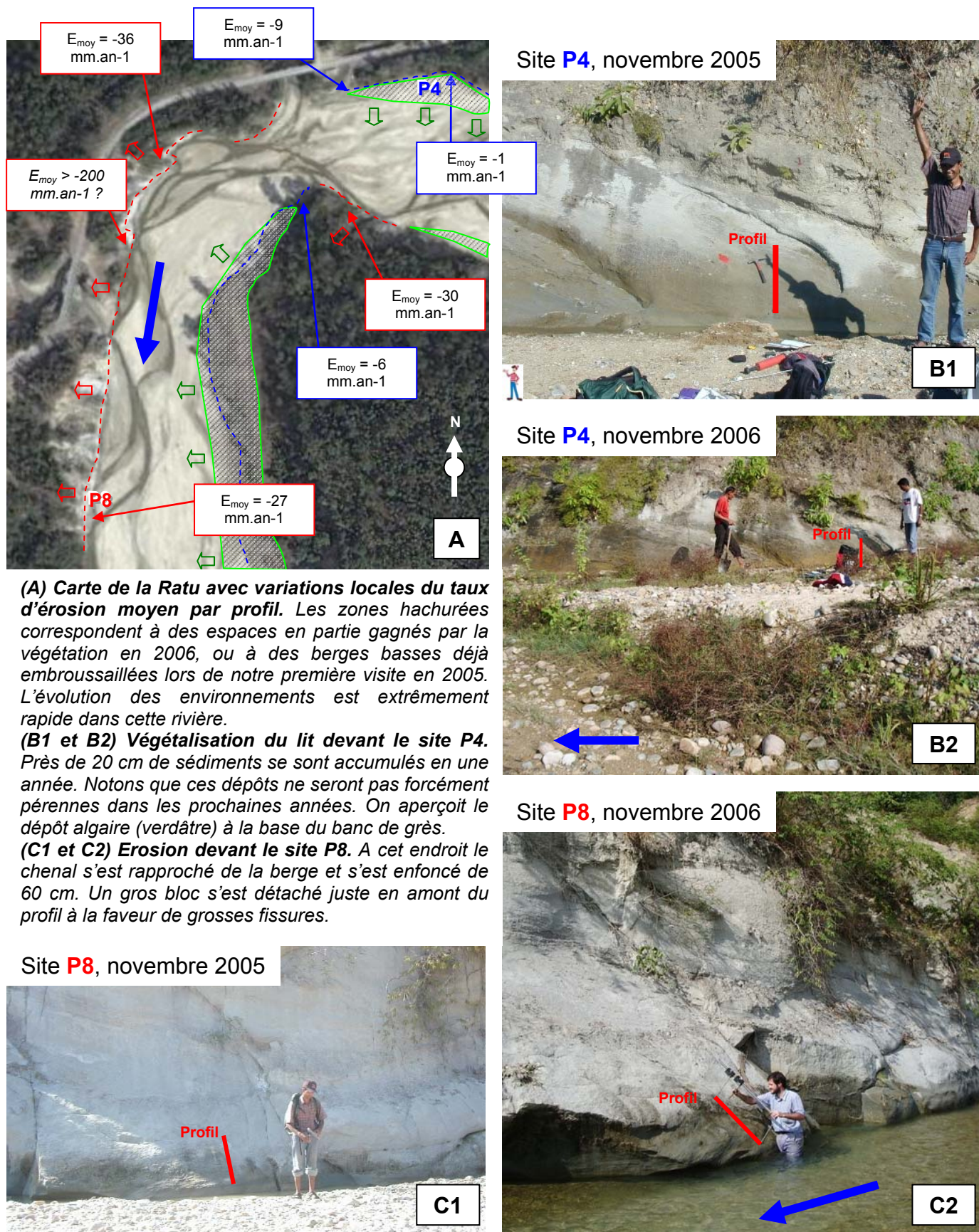
Figure 17 : Erosion en fonction de l'exposition dans le méandre de la Ratu.
