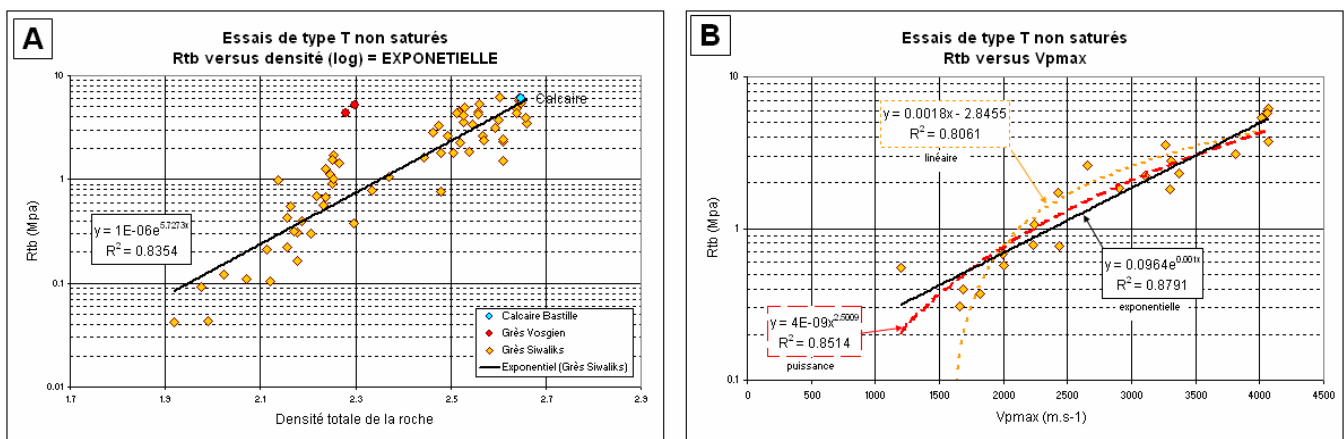
Figure 20 : Relations densité versus Rtb et vitesse des ondes P versus Rtb.
