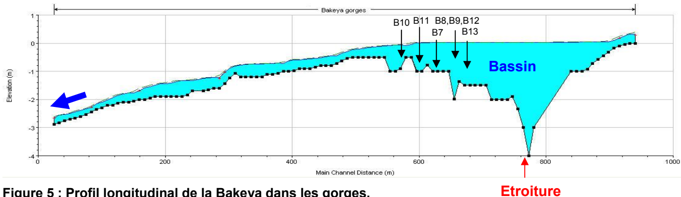
Figure 5 : Profil longitudinal de la Bakeya dans les gorges.
