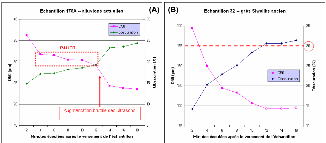
Figure 35 : Evolution du D50 et de l'obscurité dans le granulomètre laser en fonction du temps
