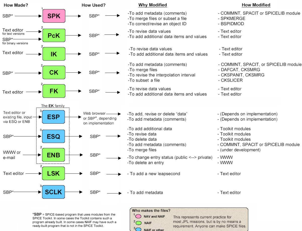
Figure B.3 – Tableau descriptif de la création et de la modification des kernels
