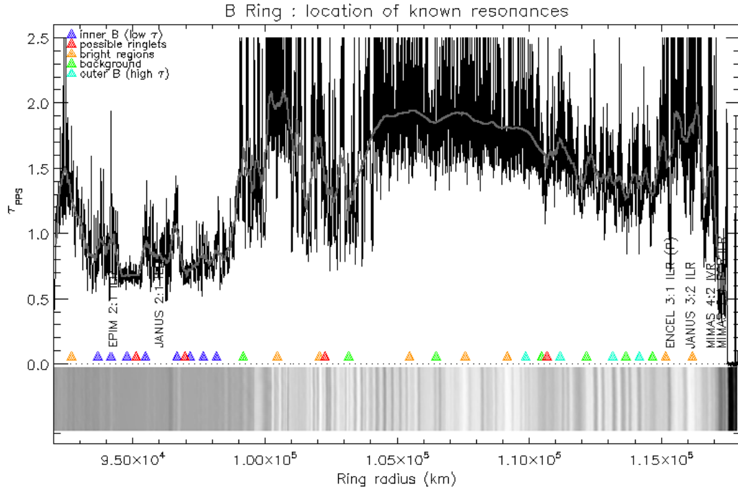
Figure D.6 – Positions théoriques des résonances dans l’anneau B, calculées par Esposito et al. (1987) et surimposées au profil de profondeur optique de l’instrument PPS de Voyager 2. La mosaïque est réalisée à partir des images Cassini N1481503960, N1481504512, N1481505090 et N1481505655 projetées dans le plan (Rayon, Longitude) des anneaux. L’angle de phase des images est de 45^\circ et la résolution radiale est de 11 \text{ km.pixel}^{-1} .
