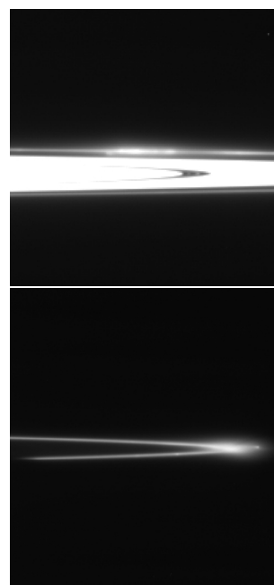
Figure 4.7 – L'anneau F vu par la tranche (images N1507015271 et N1507099722)
