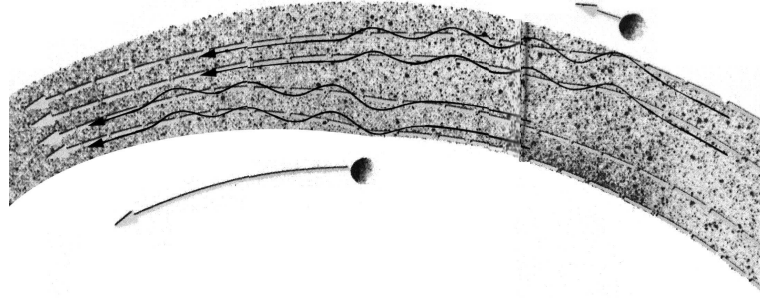
Figure 21 – Représentation schématisée de la théorie du confinement gravitationnel de Goldreich & Tremaine (1979).
