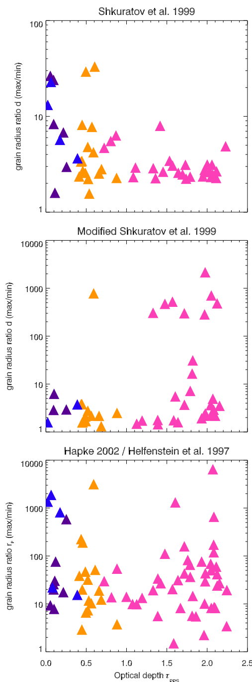
Figure 7.22 – Variation du rapport r_{\max}/r_{\min} de la taille des grains de la rétro-diffusion cohérente avec la profondeur optique.
