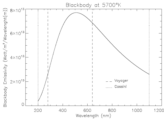
Figure 7.2 – Courbe d'émissivité de la lumière solaire, assimilée à un corps noir à 5 700 K. Les plages de longueurs d'onde de l'imageur de Voyager et de celui de Cassini sont indiquées respectivement en traits tirés et pointillés. (Mouginot, 2005)
