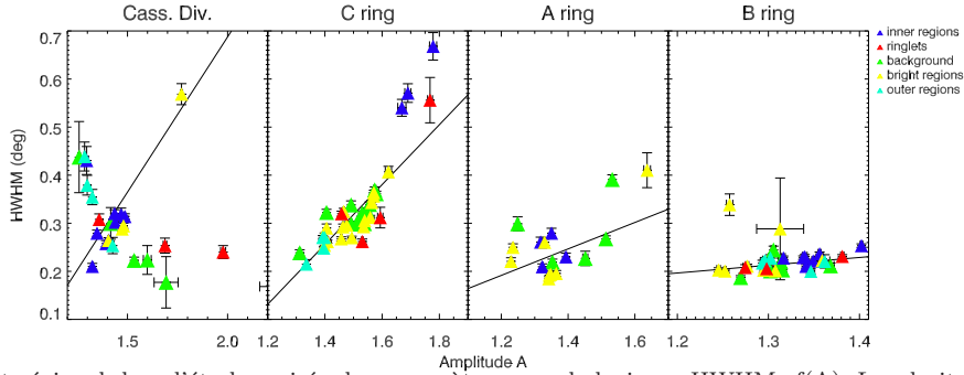
Figure G.2 – Effet régional dans l’étude croisée des paramètres morphologiques HWHM=f(A) . Les droites sont le résultat d’un ajustement linéaire donné au tableau 5.2 page 122.
