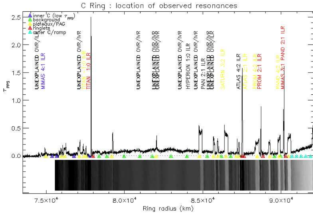
Figure D.5 – Positions théoriques des résonances dans l’anneau C, calculées par Esposito et al. (1987) et surimposées au profil de profondeur optique de l’instrument PPS de Voyager 2. Certaines ondes, assimilées à des ondes de densité par Rosen et al. (1991ab) sont également ajoutées. Deux images Cassini (N1481503400 et N1481503960) projetées dans le plan (Rayon, Longitude) des anneaux illustrent la complémentarité des images et des profils d’occultation. L’angle de phase est de 45^\circ et la résolution radiale est de 11 \text{ km.pixel}^{-1} .
