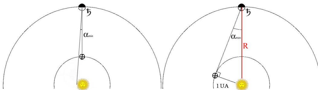
Figure 5.1 – Géométrie d'observation de l'effet d'opposition sur Terre.
