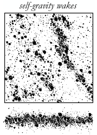
Figure 8.5 – Épaisseur d'un anneau en présence d'ondes d'instabilité gravitationnelle (Richardson, 1993).
