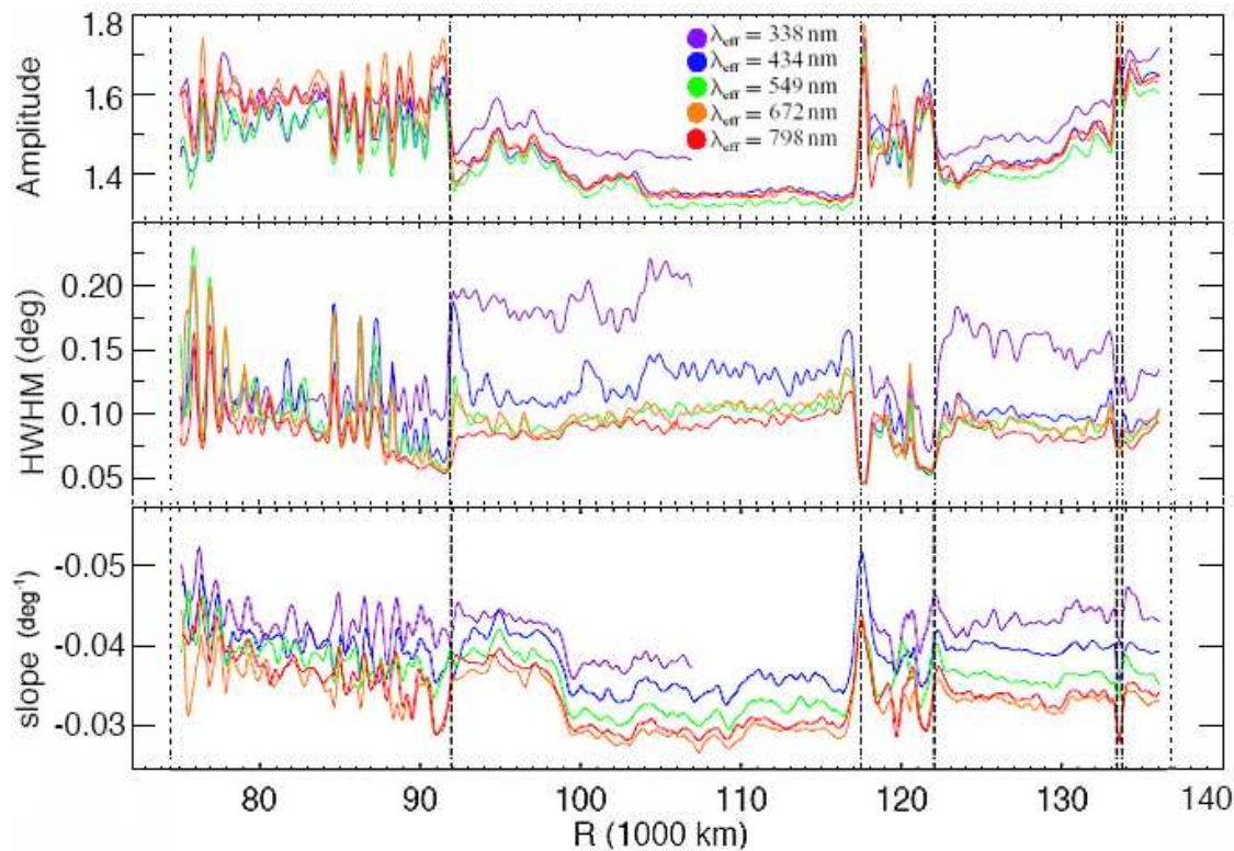
Figure 5.17 – Effet régional des paramètres morphologiques obtenus avec les courbes de phase de 0 à 6^\circ en filtres couleurs de WFPC2/Hubble à partir du modèle linéaire-exponentiel de Kaasalainen et al. (2001). Tiré de (French et al., 2007)
