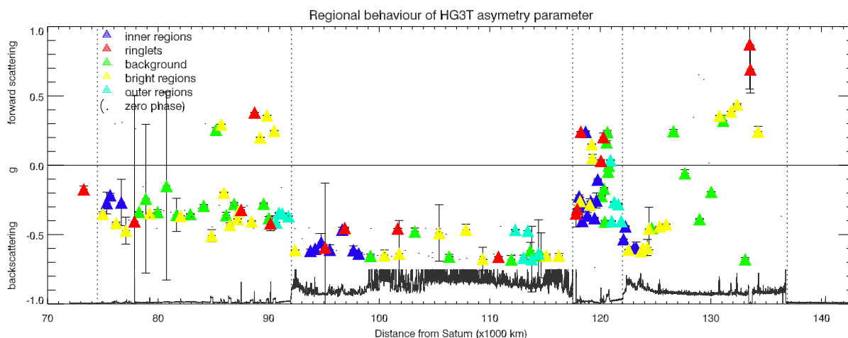
Figure G.15 – Comportement régional du paramètre d'anisotropie g obtenu par ajustement des courbes de phases en filtres CLEAR ( \lambda=611\pm 450 nm) avec le modèle de Hapke (1986) et la fonction de Henyey-Greenstein à 3 paramètres.
