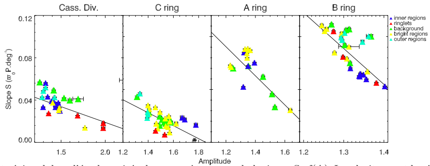
Figure G.3 – Effet régional dans l’étude croisée des paramètres morphologiques S=f(A) . Les droites sont le résultat d’un ajustement linéaire donné au tableau 5.2 page 122.
