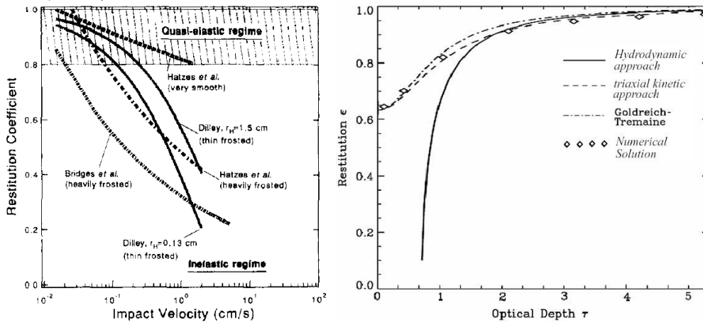
Figure 18 – Dépendance du coefficient de restitution avec la vitesse d'impact (Higa et al. , 1995) par des expériences de laboratoires et avec la profondeur optique (Schmidt et al. , 1999) en utilisant les modèles hydrodynamiques et simulations dynamiques (la relation \epsilon - \tau en traits pleins reflète une approche hydrodynamique classique; la relation \epsilon - \tau en traits pointillés équivaut à une approche cinétique triaxiale; les points tiretés se réfèrent à la formule (12) de Goldreich & Tremaine; les diamants correspondent aux simulations N-corps où la vitesse de dispersion moyenne est de l'ordre de c \sim 25\Omega_k d ( \Omega_k = \sqrt{GM}/r^3 = 1,5 \cdot 10^{-4} \text{ s}^{-1} et d = 1 \text{ m} )).
