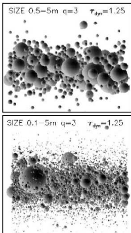
Figure 16 – Simulations dynamiques N-corps [Salo & Karjalainen, 2003]
