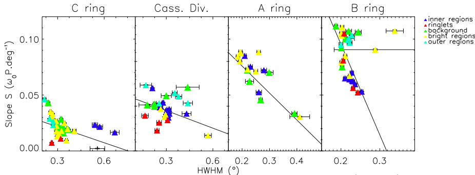
Figure G.4 – Effet régional dans l’étude croisée des paramètres morphologiques S=f(HWHM) . Les droites sont le résultat d’un ajustement linéaire donné au tableau 5.2 page 122.
