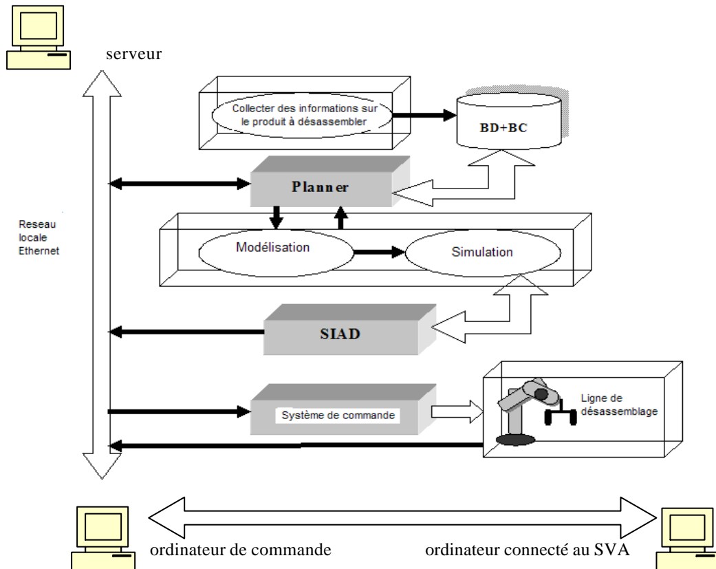
Fig. 31. Architecture du système informatique de control du désassemblage
