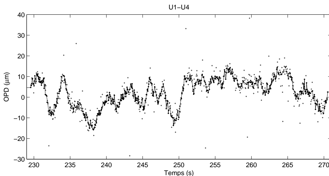
FIG. 2.6 – Exemple du filtrage par seuillage du RSB ( s = 6 ) réalisé sur la différence de chemin optique (OPD) en fonction du temps. Les points reliés par un trait plein représentent les mesures de piston différentiel ayant un RSB \geq 6 .
