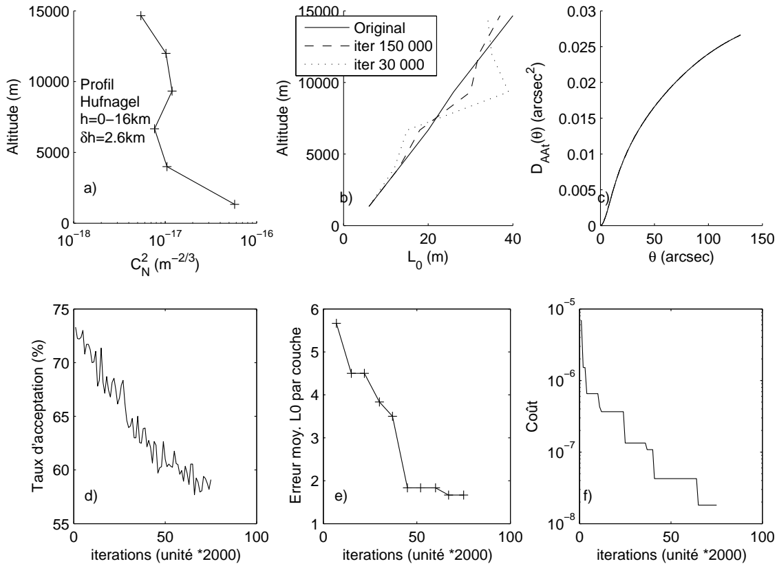
FIG. 4.12 – Exemple de reconstruction par recuit simulé d'un profil donné d'échelle externe à 6 couches d'égalles épaisseurs. a) Profil de C_N^2 utilisé suivant le modèle de Hufnagel. b) Profils d'échelle original ( trait plein ) et reconstruit pour un nombre total d'itérations donné. c) Fonction de structure angulaire des AA correspondante. d) Taux d'acceptation des perturbations générées par l'algorithme de recuit, diminuant avec la température, en fonction du nombre d'itérations. e) Erreurs moyennes sur les valeurs d'échelle obtenues par couche équivalente (Eq.4.12). f) Fonction de coût correspondante représentée à chaque changement de température (2000 itérations à T constant).
