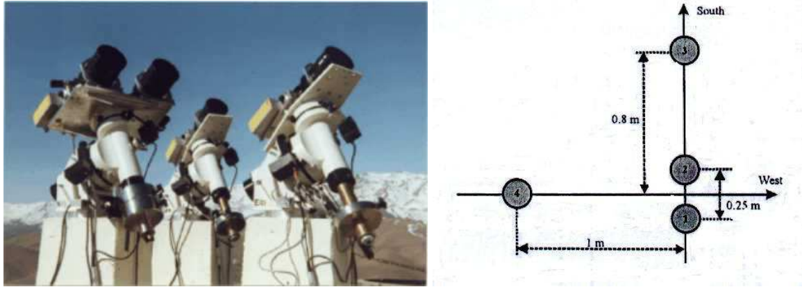
FIG. 1.9 – Photo du Generalized Seeing Monitor (GSM) et représentation de sa configuration standard à 4 télescopes (F. Martin et al 1998 [94], A. Ziad et al 2000 [171]). Il permet d’effectuer une analyse statistique des fluctuations d’AA pour déterminer les paramètres optiques de la turbulence atmosphérique.
