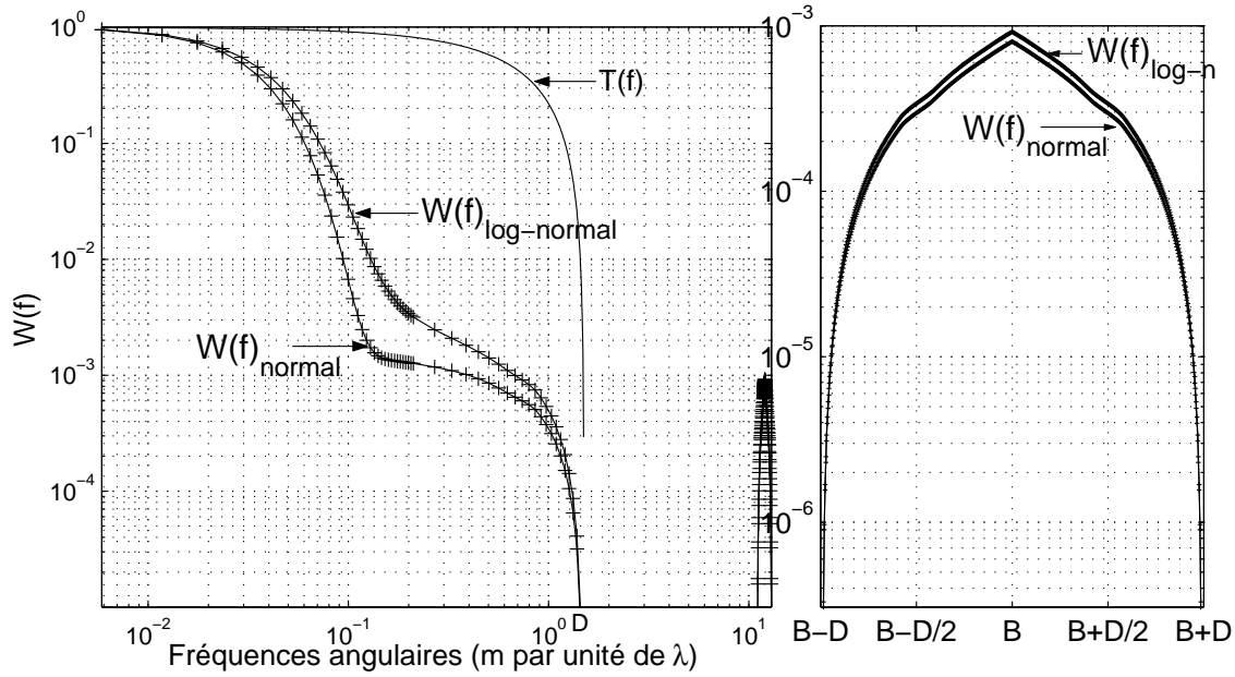
FIG. 2.12 – Densités spectrales W(\vec{f})^{log-normal} et W(\vec{f})^{normal} calculées pour B = 12m , D = 1.5m (cas du GI2T), D_{Obs} = 0.15D , r_0 = 12cm dans le cas du modèle de turbulence de Kolmogorov. Les pics franges sont représentés sur la partie droite.
