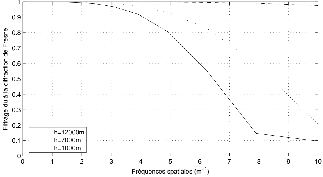
FIG. 3.5 – Filtrage dû à la propagation de Fresnel pour différentes altitudes des couches turbulentes ( \lambda = 0.5\mu\text{m} ).
