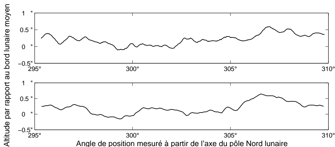
FIG. 4.9 – Comparaison du bord moyen mesuré ( haut ) le 17 Juillet 2005 (08h19'TU) à Mauna Kea et profil de Watts correspondant ( bas ) où la libration en longitude est l = -7.4^\circ et en latitude b = 4.6^\circ .
