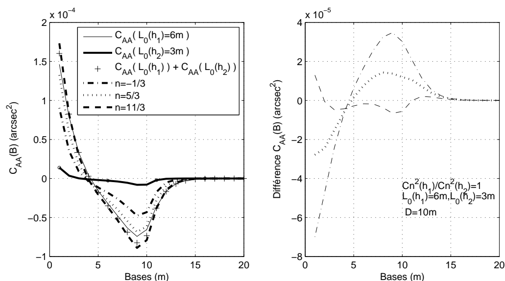
FIG. 3.8 – Somme des covariances longitudinales des fluctuations d'AA pour \mathcal{L}_0(h_1) = 6\text{m} et \mathcal{L}_0(h_2) = 3\text{m} avec D = 10\text{m} (à gauche). Erreur absolue associée à l'ajustement par des covariances calculées en utilisant une échelle externe déduite de l'Eq.3.10. Dans ce cas, l'erreur est minimale lorsque n = 11/3 .
