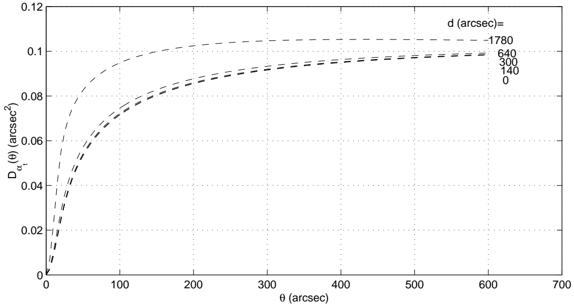
FIG. 4.8 – Effet maximal de la courbure du bord de la Lune sur les fonctions de structure des AA pour différentes distances de bord d = 0, 140, 300, 640 et 1780 \text{arcsec} correspondant respectivement à \gamma = 90, 85, 80, 69 et 0^\circ lorsque r_0 = 0.15m , \mathcal{L}_0 = 25m , h = 2000m et D = 0.2m .
