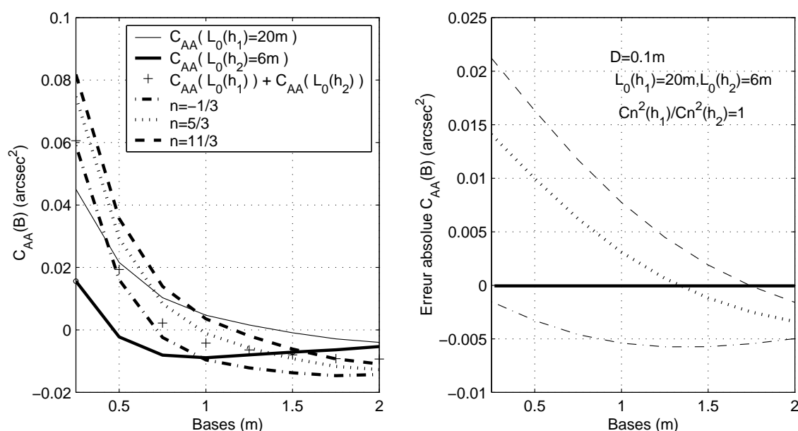
FIG. 3.9 – Somme des covariances longitudinales des fluctuations d'AA pour \mathcal{L}_0(h_1) = 20\text{m} et \mathcal{L}_0(h_2) = 6\text{m} avec D = 0.1\text{m} (à gauche). Erreur absolue associée à l'ajustement par des covariances calculées en utilisant une échelle externe déduite de l'Eq.3.10. Dans ce cas, la valeur de n pour laquelle l'erreur est minimale dépend de la base.
