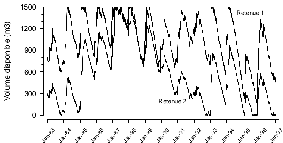
Figure 10. Simulation des stocks disponibles dans une retenue collinaire individuelle : comparaison du système de collecte de ruissellement actuel, et d'un système amélioré. (simulation sur série de données climatiques pluriannuelles)
