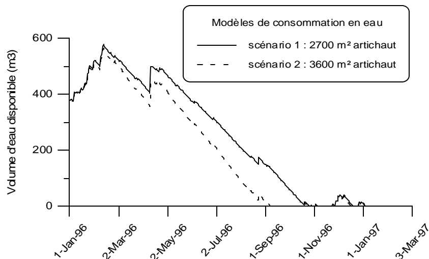
Figure 9. Simulation du stock disponible dans une retenue collinaire individuelle, selon la surface en une culture donnée et fonction des consommations (basées sur les modèles d'action) (simulation sur les données climatiques d'une année sèche –quartile-)
