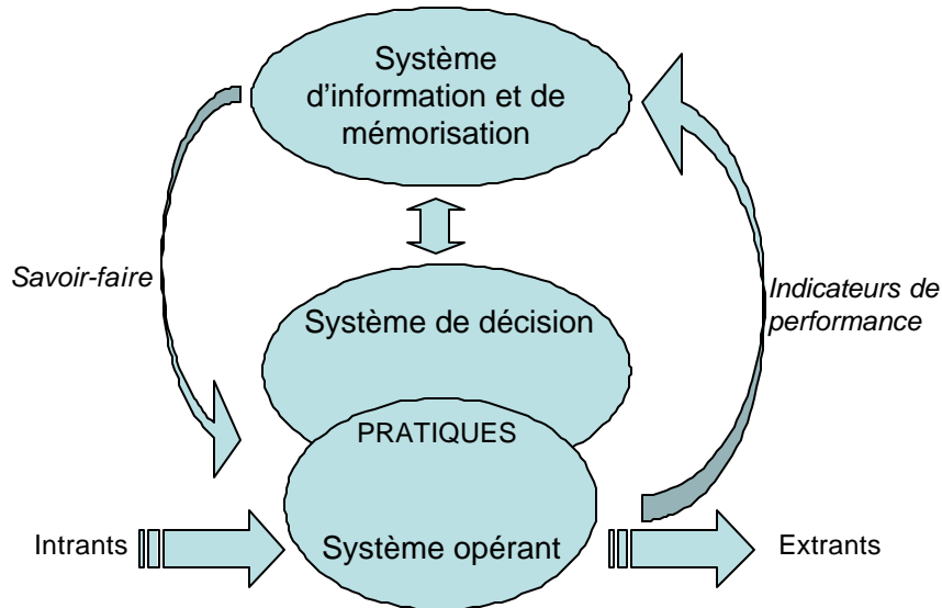
Figure 6. Articulation entre système d'information, système de décision et système opérant dans l'exploitation agricole. Localisation des pratiques (adapté de Landais & Deffontaines, 1988, et 105)
