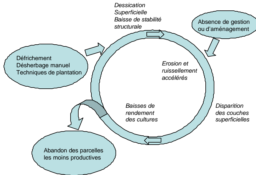
Figure 3. Modèle d'évolution des horizons superficiels des andosols sous systèmes à base de géranium à la Réunion : interactions entre pratiques culturales et état du sol (5).
