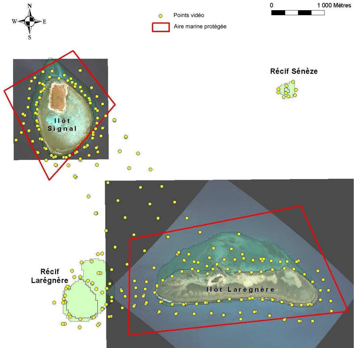
Figure 5.10 (adaptée de Pelletier & Leleu 2008) : Plan d'échantillonnage par station vidéo rotative pour la zone du lagon sud-ouest (ilots Signal et Larégnère), en juin-juillet 2007.
