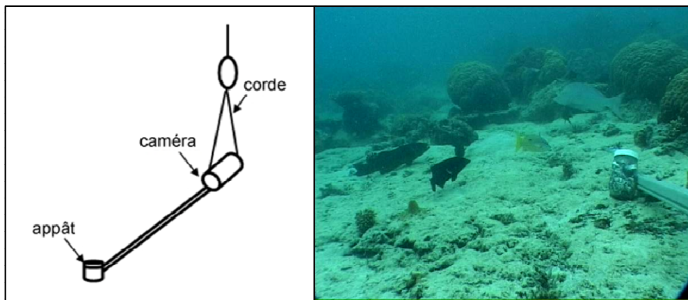
Figure 5.7 : Dispositif de vidéo appâtée et capture d'écran d'une vidéo en cours d'échantillonnage (Photo : Tim Langlois).
