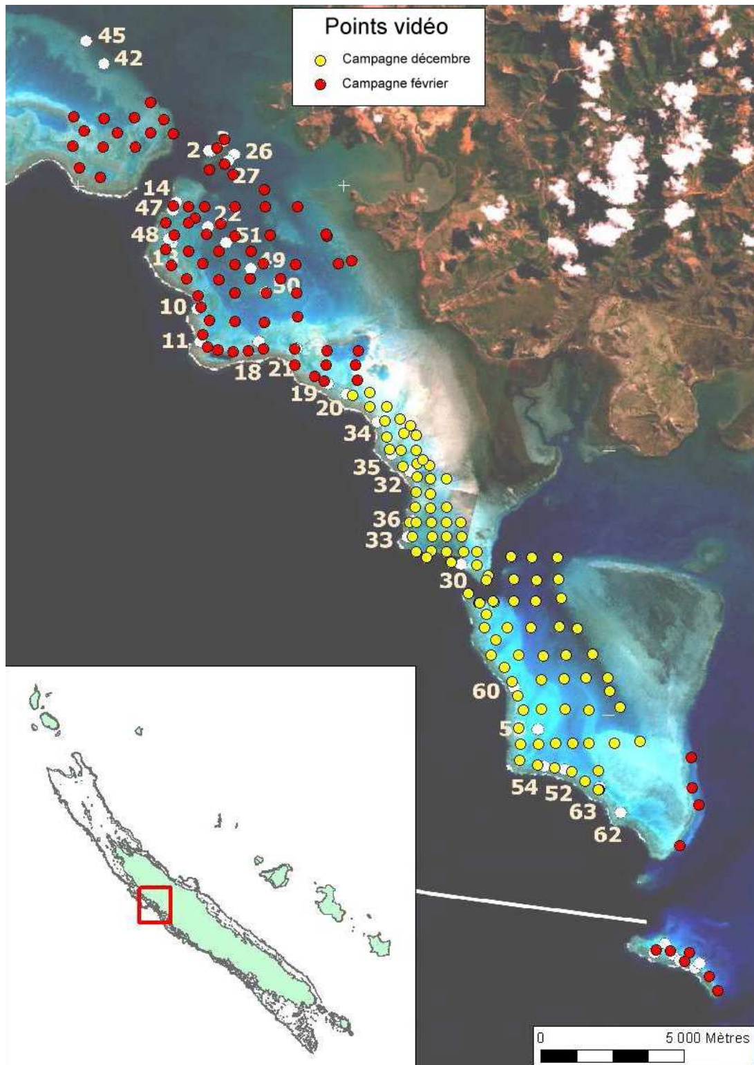
Figure 5.11 (adaptée de Pelletier & Leleu 2008): Plan d'échantillonnage par station vidéo rotative pour la zone VKP, en décembre 2007 et février 2008.
