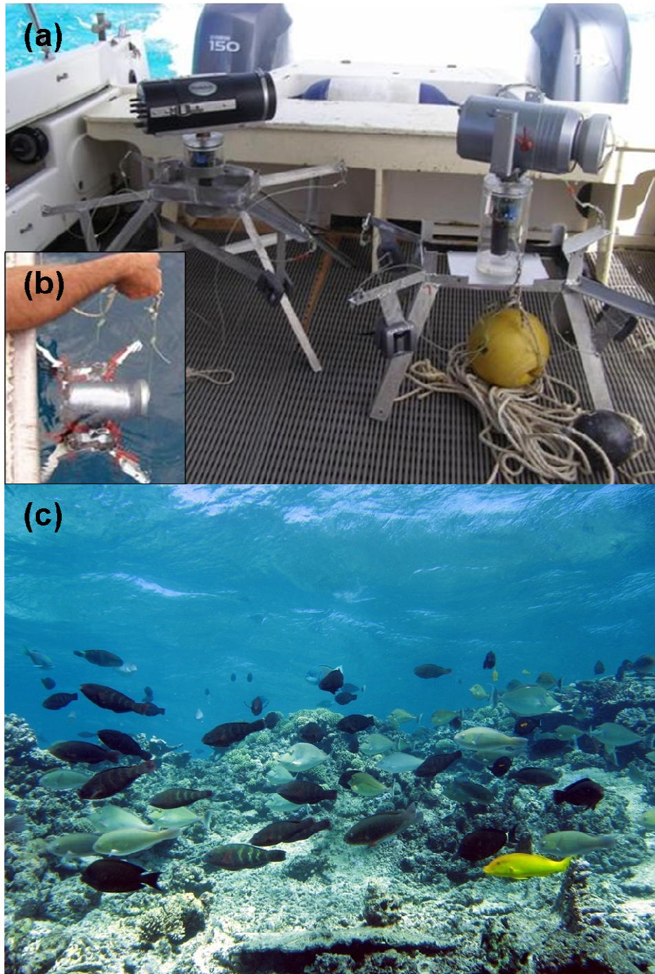
Figure 5.9 : (a) Systèmes vidéo rotatifs utilisés lors de l'échantillonnage des zones lagon sud-ouest et VKP ; (b) mise à l'eau d'un système ; (c) capture d'écran d'une séquence vidéo lors d'un échantillonnage (Photos : Kevin Leleu, Dominique Pelletier).
