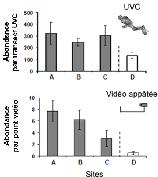
Figure 5.8 (adaptée de Langlois et al. 2006) : Comparaison des abondances observées par UVC et par vidéo appâtée, respectivement pour un transect de 50m et un point vidéo (2 répliquats dans chaque cas). Sites A, B, C : aire marine protégée ; site D : site non-protégé.
