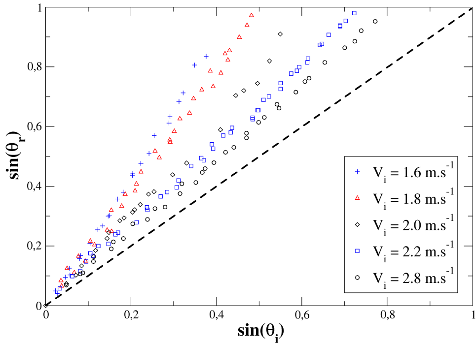
FIGURE 2.20 – Sinus de l’angle d’incidence du jet entrant en fonction du sinus de l’angle du jet sortant pour un rayon de jet entrant R_i = 80 \text{ } \mu\text{m} et pour différentes vitesses. En pointillés : \sin(\theta_i) = \sin(\theta_r)
