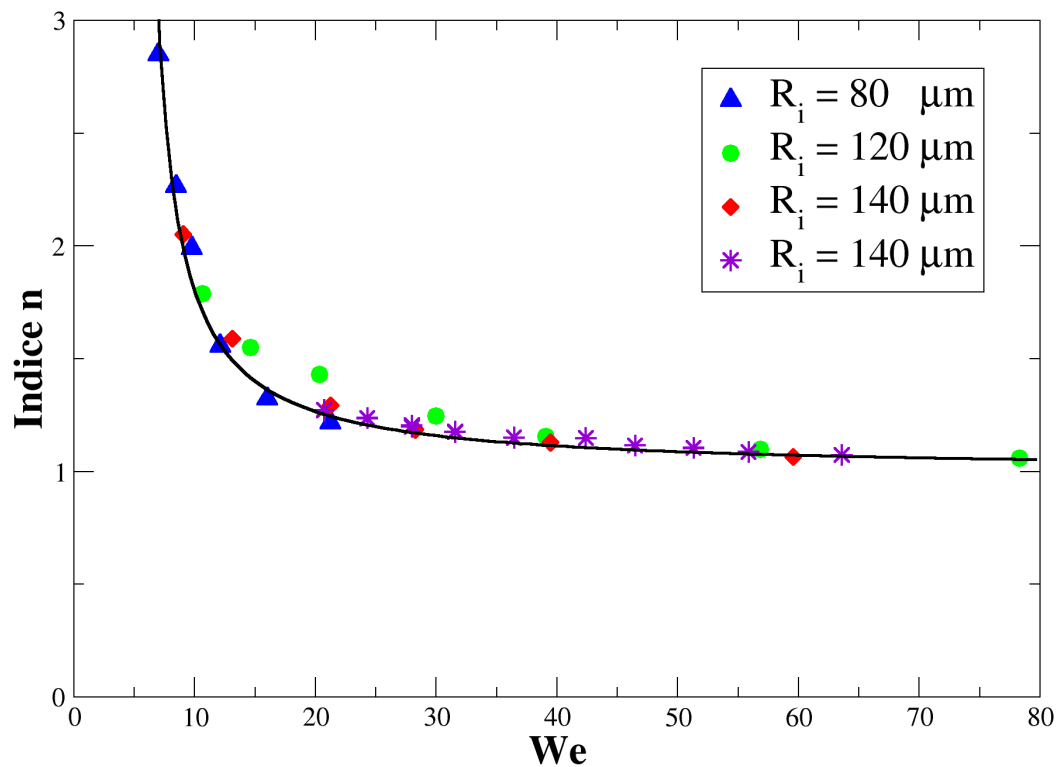
FIGURE 2.22 – Indice de réfraction n en fonction du nombre de Weber pour différentes vitesses, trois rayons de jet différents et deux solutions différentes : R_i = 80 \mu m (▲), 120 \mu m (●), et 140 \mu m (◆) pour la solution de Dreft, et R_i = 140 \mu m pour la solution de TTAB (*). En trait plein noir, la courbe de l'équation 2.22 .
