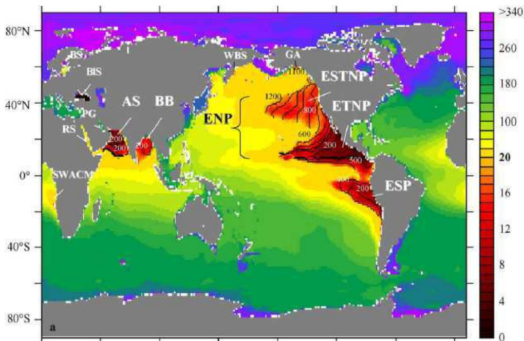
Figure 1.23: Distribution de l'oxygène ( \mu M \equiv mmolO_2.m^{-3} ) en profondeur, au niveau du minimum d'oxygène, indiquant l'étendue des OMZs (en rouge) selon la climatologie
