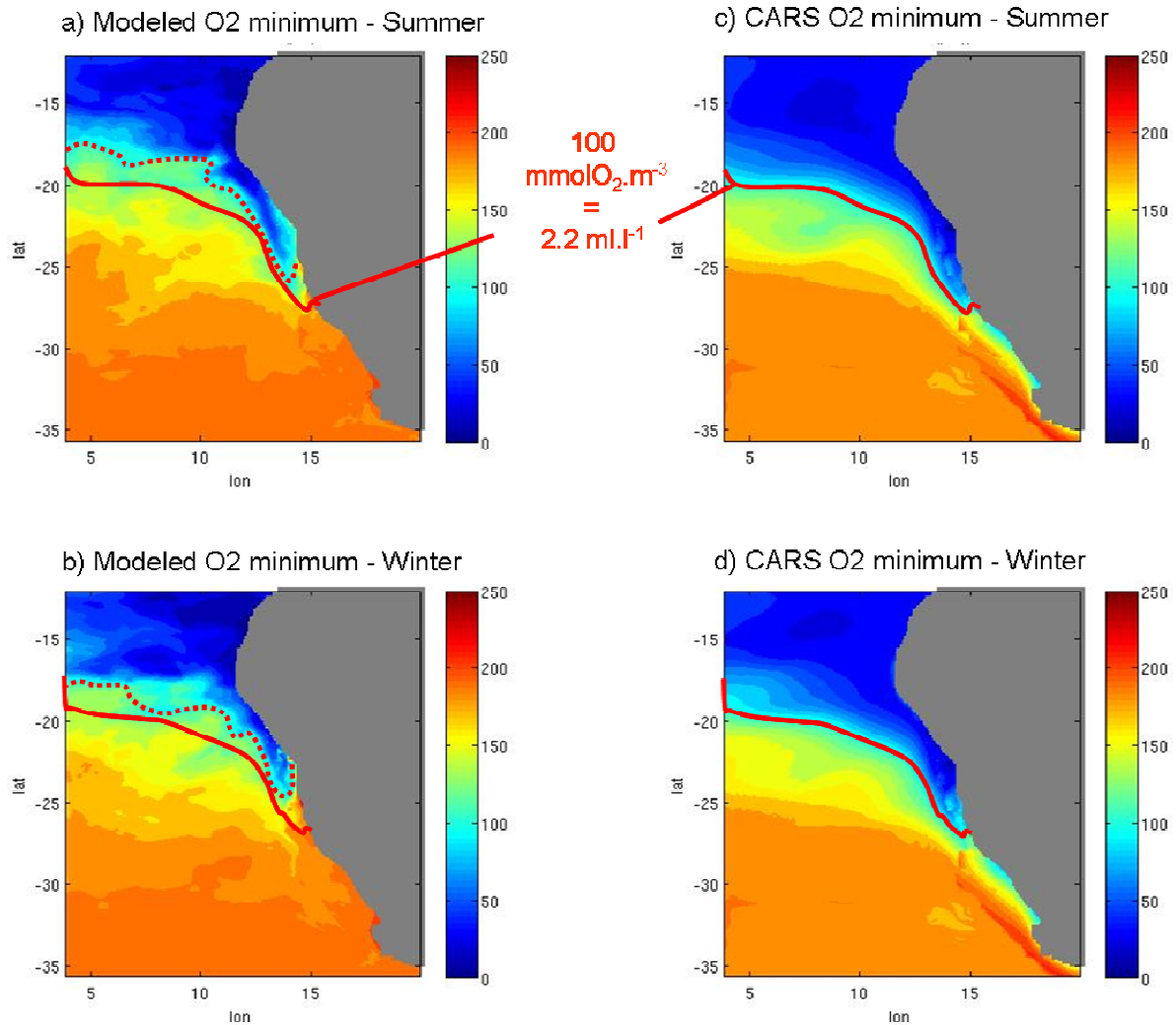
Figure 1: Minimum d'oxygène (mmolO 2 .m -3 ) simulé par le modèle couplé ROMS-BioSUS en configuration SAfE en été (a) et en hiver (b) et minimum d'oxygène issu des données mensuelles de la climatologie CARS en été (c) et en hiver (d).
