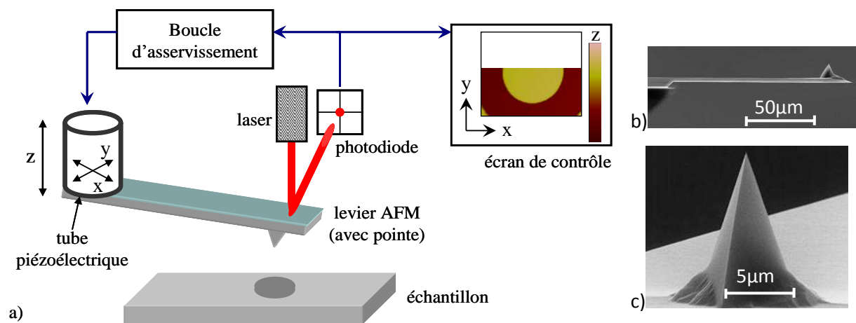
Figure 59 : a) Principe de l'AFM, b) et c) exemples de levier et pointe AFM [NanoW]
