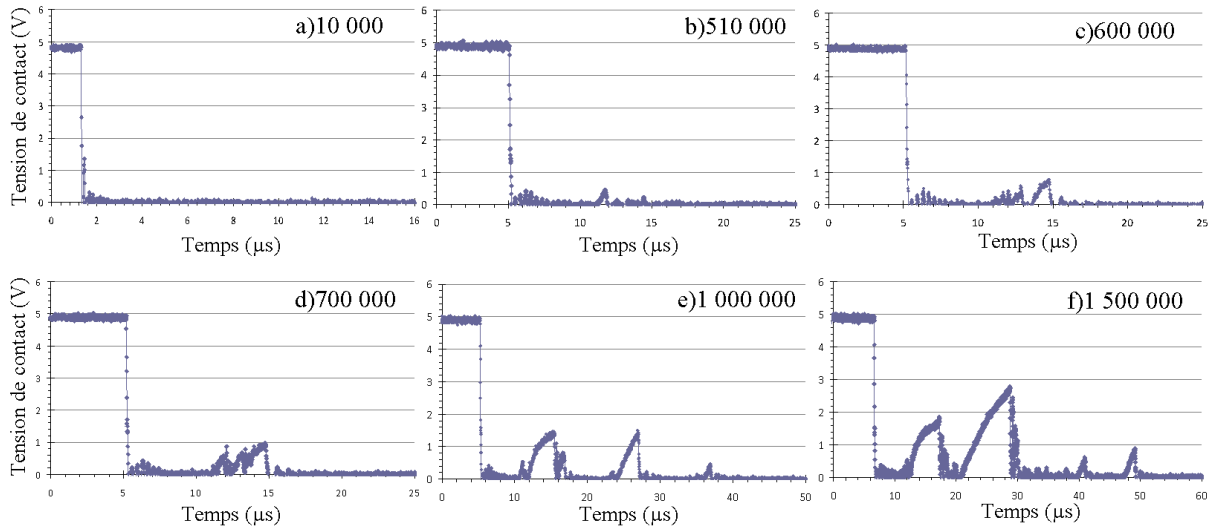
Figure 137 : Evolution de la tension de contact à la fermeture du relais Omron-1 pour a) 10000, b) 510000, c) 600000, d) 700000, e) 1000000 et f) 1500000 cycles (f=2Hz, 5V/500μA)
