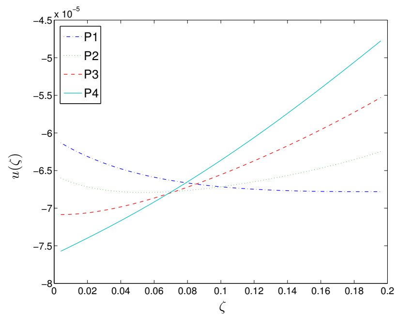
FIGURE 4.15 – Dépendance en \zeta de la composante u du déplacement pour les trois points définis sur la figure 4.14
