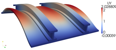
FIGURE 3.8 – Déformée de la plaque raidie
