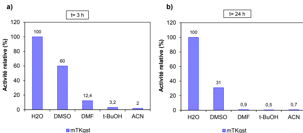
Figure 50 : Activités résiduelles de mTK gst après incubation dans 50% de cosolvant à 50 °C
