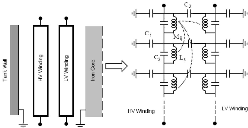
Figure 36 : Modélisation d'un transformateur en self et capacités
