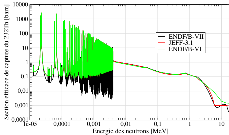
FIGURE 2.8: Sections efficaces neutroniques de capture (n,γ) du ^{232}\text{Th} extraits des bases ENDF/B-VI, ENDF/B-VII.1 et JEFF-3.1
