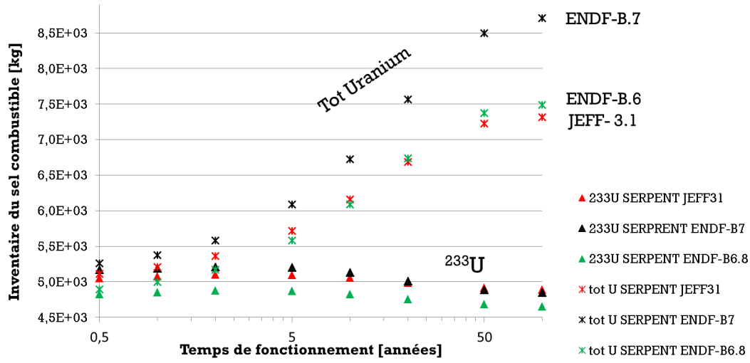
FIGURE 2.35: Évolution de l'inventaire du sel combustible en uranium et en ^{233}\text{U} des évaluations de POLIMI (SERPENT) utilisant trois différentes bases de données ENDF-B.VI, ENDF-B.VII et JEFF-3.1
