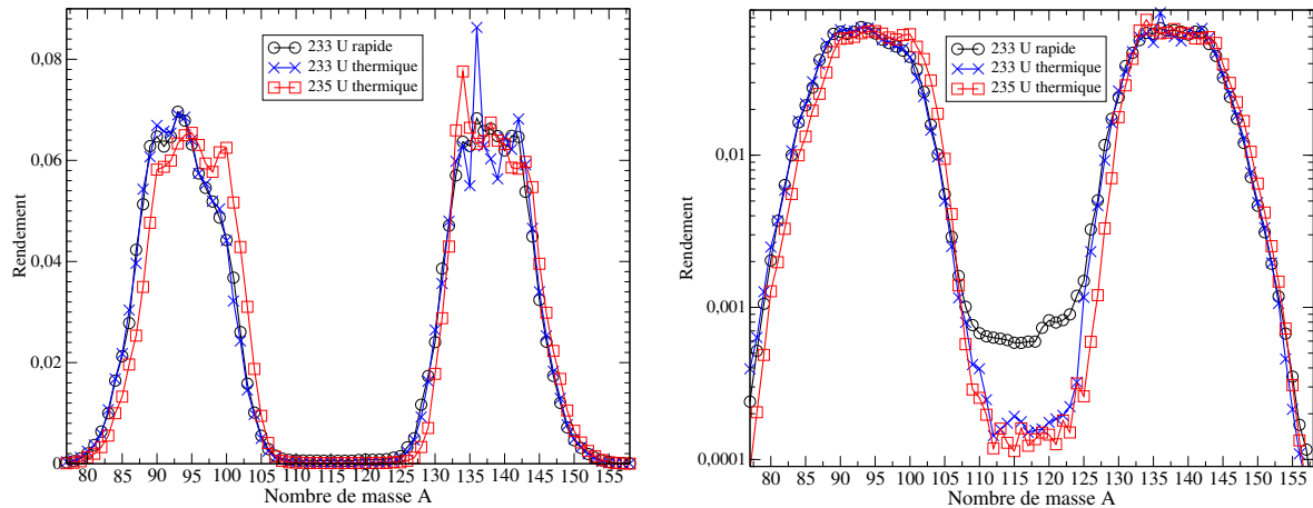
FIGURE 4.4: Distribution des fragments de fission en fonction de leur nombre de masse A pour ^{235}\text{U} en spectre thermique ( \langle E_{\text{neutron}} \rangle = 0,0235 eV, en rouge) et ^{233}\text{U} en spectres rapide ( \langle E_{\text{neutron}} \rangle = 500 keV, en noir) et thermique (en bleu); à gauche en représentation linéaire - à droite en représentation logarithmique; base de données des rendements de fission : JEFF-3.1.1
