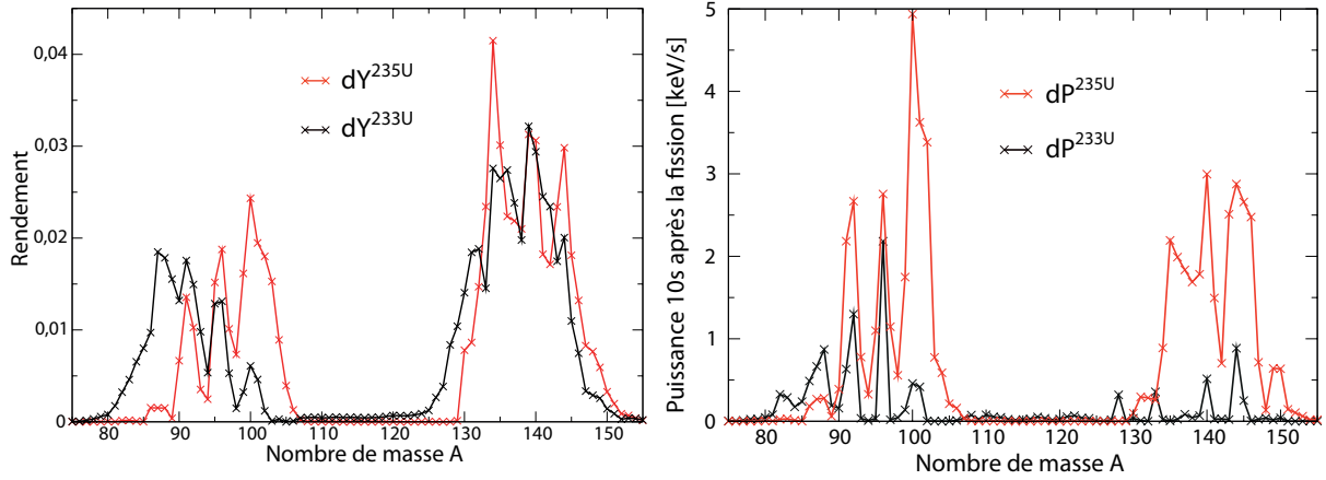
FIGURE 4.7: À gauche : Différence des rendements de fission dY_i de ^{235}\text{U} en spectre thermique et de ^{233}\text{U} en spectre rapide en fonction du nombre atomique A ; à droite : Puissance émise 10 s après la fission par les vecteurs isotopiques des différences de rendements de fission de ^{233}\text{U} en spectre rapide et ^{235}\text{U} en spectre thermique respectivement dY_i^{235U} et dY_i^{233U} , en fonction du nombre atomique A
