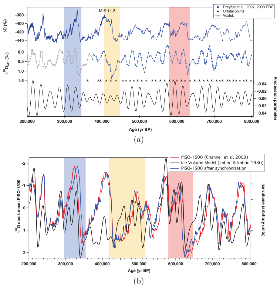
FIGURE 6.9 – (a) Données de \delta^{18}\text{O}_{\text{atm}} (marqueurs bleus) mesurées sur la carotte de glace EDC [Dreyfus et al., 2007] alignées sur le signal de précession décalé 5000 ans plus jeune (courbe noire) [Laskar et al., 2004] pour la construction de la chronologie EDC3 [Parrenin et al., 2007b]. Des mesures de \delta^{18}\text{O}_{\text{atm}} de Vostok sur l'échelle d'âge EDC3 sont incluses pour comparaison (marqueurs gris, non publiés). (b) \delta^{18}\text{O} marin de PISO-1500 avant (rouge) et après synchronisation (bleu) de son signal paléomagnétique sur le flux de ^{10}\text{Be} à EDC, et sortie du modèle de volume de glace (courbe noire, basée sur l'insolation du 21 Juin à 65^\circ\text{N} , [Imbrie and Imbrie, 1980]) utilisée pour la construction de la chronologie de composite de \delta^{18}\text{O} benthique LR04 [Lisiecki and Raymo, 2005]. La zone jaune souligne l'intervalle de temps où l'alignement orbital est le moins certain (voir texte et section 6.3.2 pour les zones bleues et rouges).
