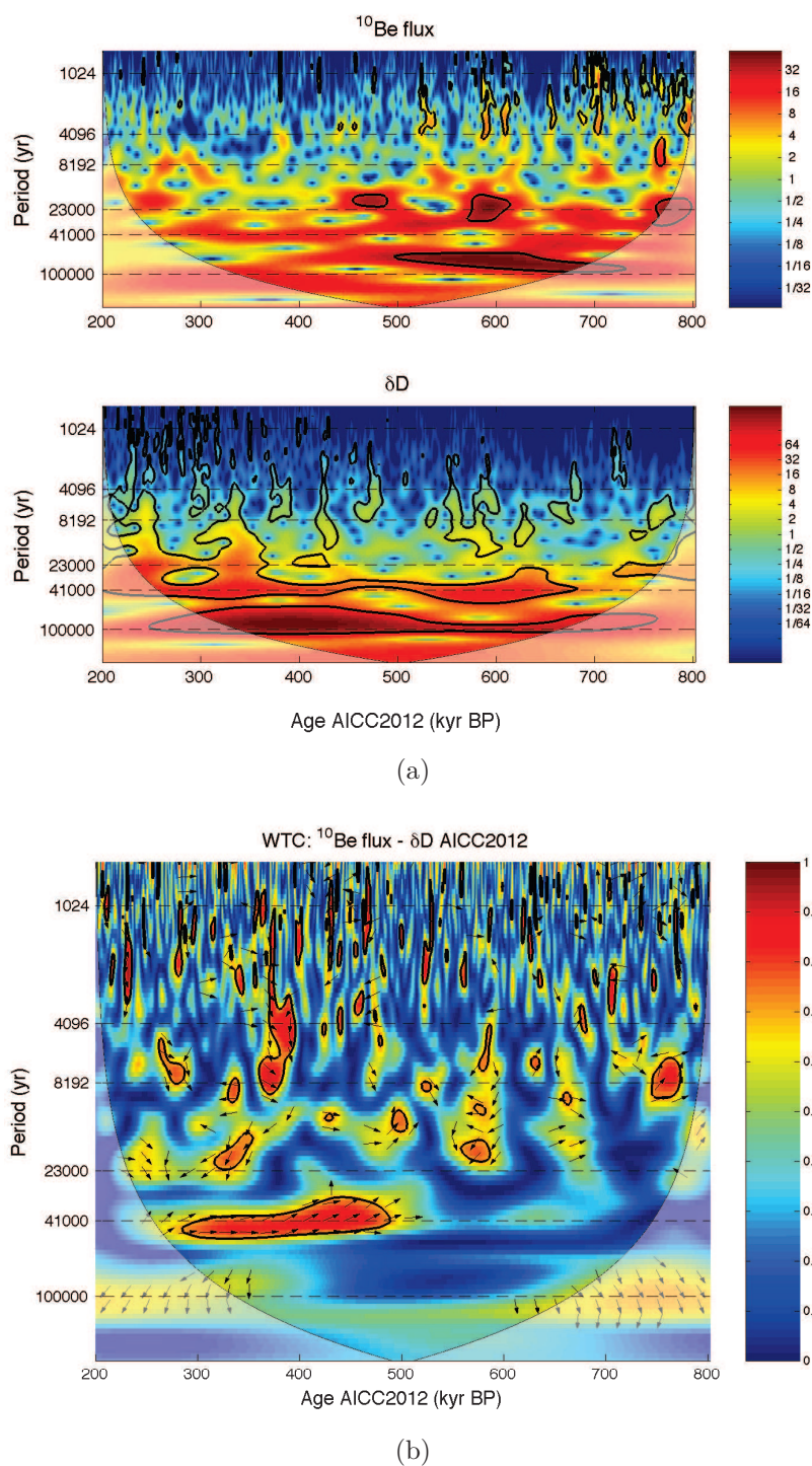
FIGURE D.2 – (a) Analyse en ondelettes du flux de ^{10}\text{Be} et du \delta\text{D} et (b) carte de corrélation locale (WTC) dans l'espace temps – fréquence entre les deux spectres sur l'échelle d'âge AICC2012 [Bazin et al., 2013].
