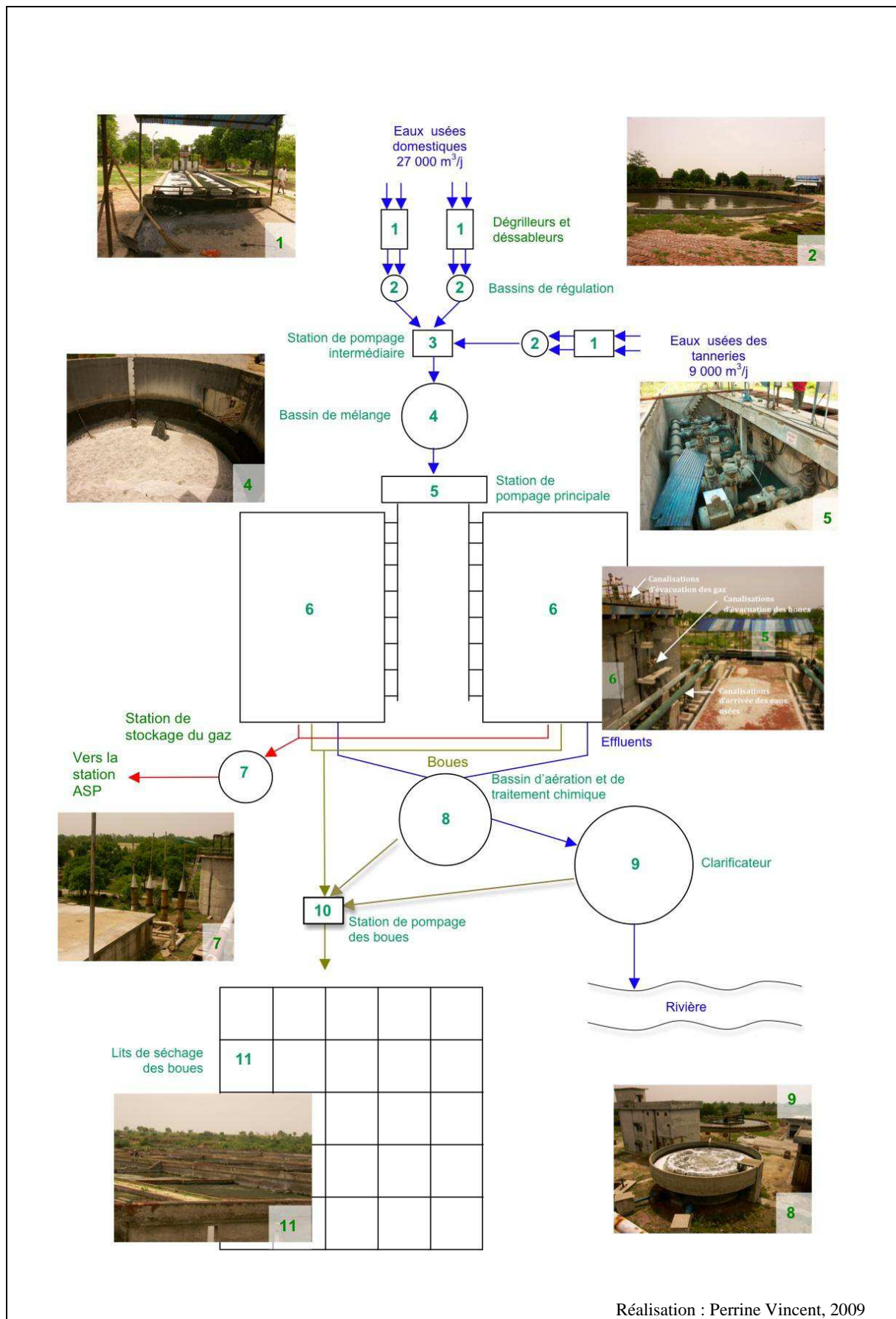
Schéma 4 – la station UASB de 36 000 m³/j et le post traitement, Kanpur
