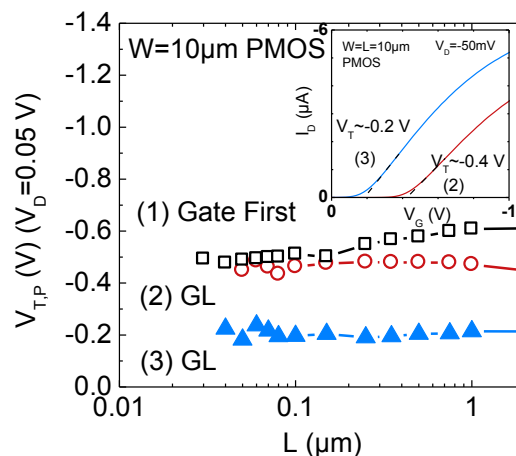
Figure III.27: Tension de seuil ( V_T ) à V_D = -50 mV sur des pFET large ( W = 10 \mu\text{m} ) en fonction de la longueur de grille.
