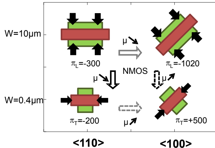
Figure II.44: Schéma des zones actives de nFET larges ( W=10\mu\text{m} ) et étroits ( W=0.4\mu\text{m} ). Les flèches noires représentent la contrainte compressive longitudinale ou transverse induite par le STI ainsi que les coefficients piézorésistifs associés ( 10^{-12}.\text{Pa}^{-1} ) [Dorda71]. (une contrainte compressive associée à un coefficient négatif dégrade la mobilité)
