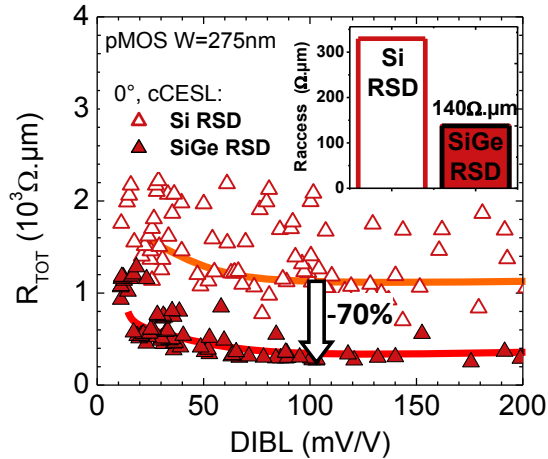
Figure III.34: Effet des S/D SiGe comparé aux S/D Si sur la résistance totale ( R_{TOT} ) en fonction du DIBL pour des pFET selon \langle 110 \rangle / (001) avec un CESL compressif.
