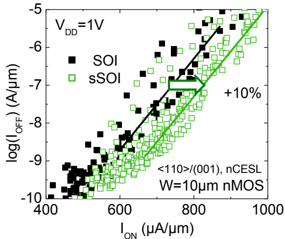
Figure II.26: Compromis I_{ON} - I_{OFF} des nFET ( L_{nom}=35 nm, W=10 µm) sur SOI et sSOI.
