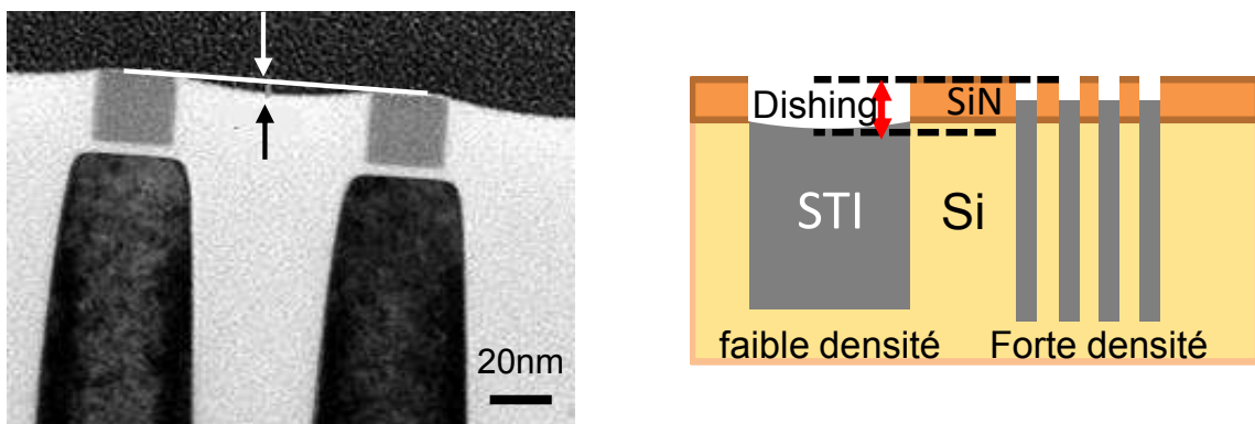
Figure III.12 : Image TEM et schéma du dishing du STI.
