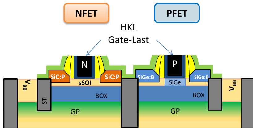
Figure IV.37: Schéma d'intégration CMOS proposé pour le nœud technologique 10 nm sur SOI.
