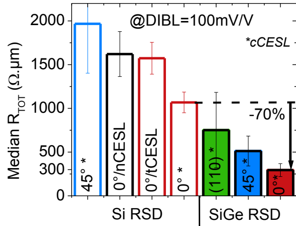
Figure III.35: R_{TOT} médian de pFET GL avec différentes configurations de surfaces/orientation et S/D à un DIBL de 100mV/V.
