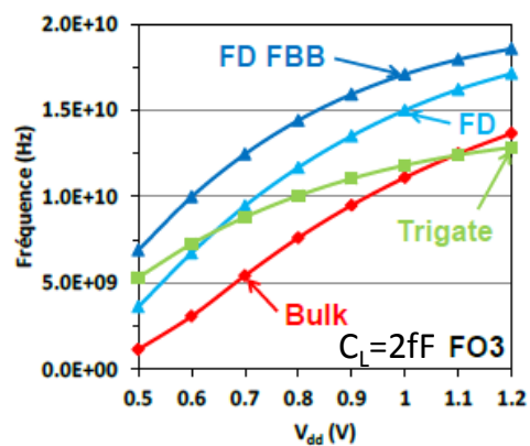
Figure I.15: Simulations de la fréquence d'un oscillateur en anneau en fonction de la tension d'alimentation pour différentes architectures au nœud 14 nm [Lacord13].
