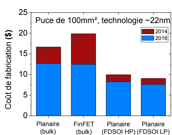
Figure I.5: Estimation du coût de fabrication d'une puce de 100mm² pour différentes architectures [IBS12].
