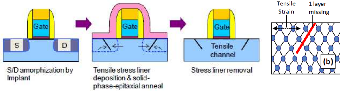
Figure II.6: Schémas de l'enchaînement des étapes permettant de créer des dislocations par SMT dans les S/D [Lim10].
