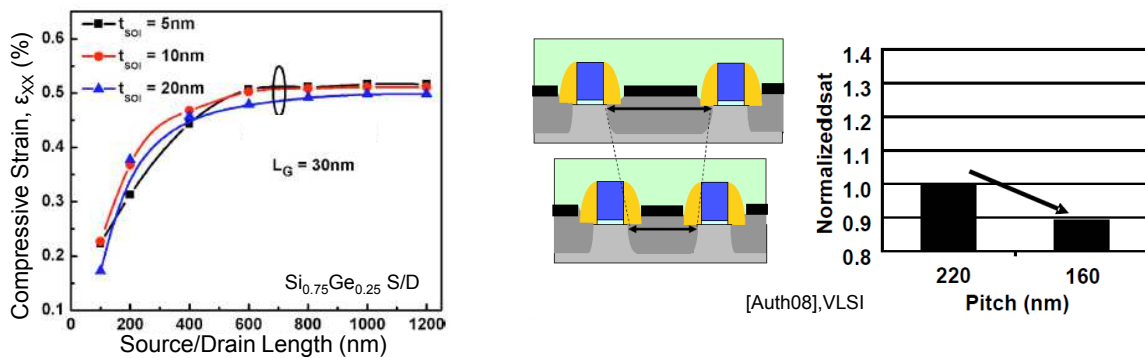
Figure II.39: Diminution de la contrainte dans le canal [Madan08] et du gain en courant [Kuhn09] avec la diminution de l'espace entre les grilles avec des S/D en SiGe
