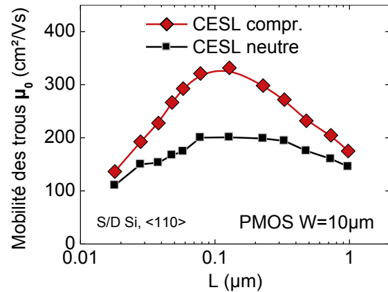
Figure II.21: Mobilité à faible champ des trous sur des pFET selon \langle 110 \rangle avec un CESL neutre ou compressif.
