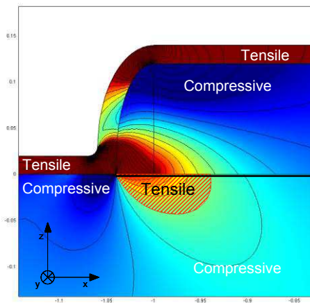
Figure II.11: Déformation longitudinale ( \sigma_{xx} ) due à un CESL tensile sur un transistor bulk [Payet08t].
