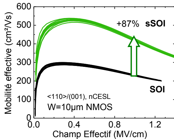
Figure II.28: Mobilité effective des électrons en fonction du champ effectif pour des nFET longs et larges ( L=10 µm, W=10 µm).
