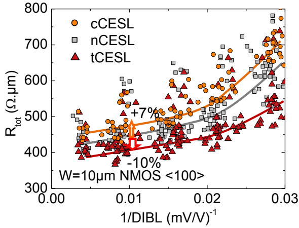
Figure II.15: R_{TOT} en fonction de 1/DIBL pour des nFET selon \langle 100 \rangle avec différents CESL à W=10 \mu\text{m} et L < 90 \text{ nm} .
