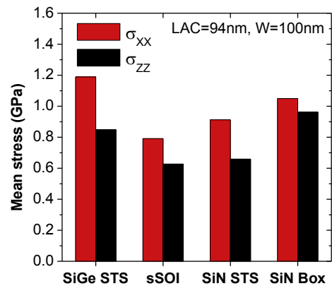
Figure IV.13: Valeur moyenne dans le silicium et schémas des structures simulées : SiGe STS, sSOI, SiN STS et BOX contraint.
