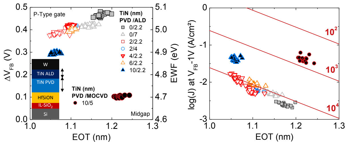
Figure III.16 : Décalage de la tension de bande plate par rapport au midgap ( \Delta V_{FB} ) et courant de fuite (à droite) en fonction de l'EOT pour différent contact de grille sur des MOSCAP HKF-GL
