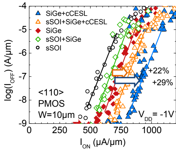
Figure II.22: I_{ON}-I_{OFF} de pFET gate-first sur SOI avec différentes configurations intégrant de la contrainte par un substrat sSOI, S/D SiGe:B ou cCESL. ( W=10\mu\text{m} , L_{nom}=35-45\text{ nm} ) (procédés par défaut : SOI, S/D Si, nCESL)
