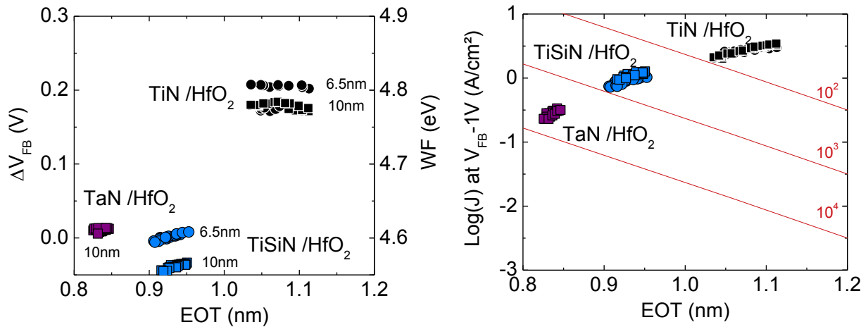
Figure III.41: Décalage de la tension de bande plate par rapport au midgap ( \Delta V_{FB} ) et courant de fuite (à droite) en fonction de l'EOT pour différents empilements de grille sur des MOSCAP avec HfO 2 non recuit (type HKL).
