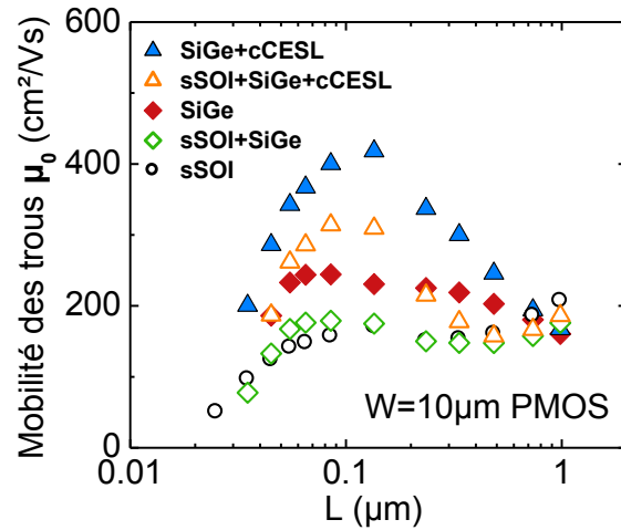
Figure II.23: Mobilité à faible champ des trous sur des pFET sur SOI avec différentes configurations intégrant de la contrainte par un substrat sSOI, S/D SiGe:B ou cCESL.
