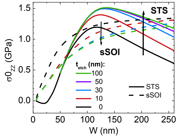
Figure IV.4: Influence de la sur gravure dans le silicium sur la contrainte au centre de la zone active ( \sigma_{zz} ) en fonction de W pour le STS et le sSOI.
