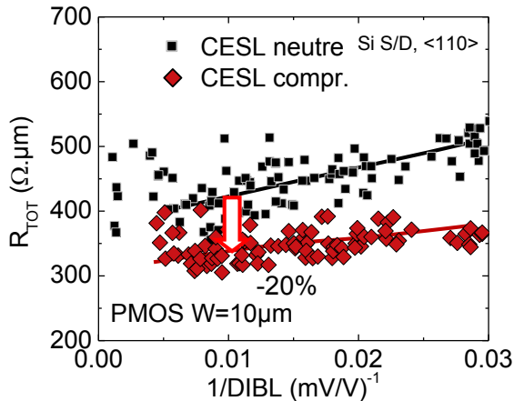
Figure II.20: R_{TOT} en fonction du DIBL pour des pFET selon \langle 110 \rangle avec un CESL neutre ou compressif ( W=10\ \mu\text{m} et L<90\ \text{nm} ).
