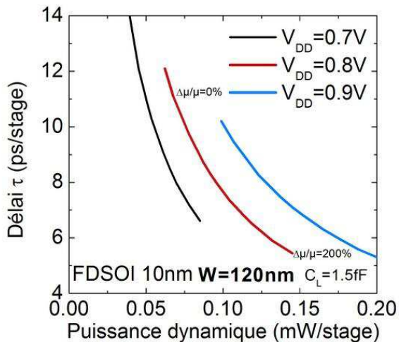
Figure IV.33: Simulation du délai en fonction de la puissance dynamique d'un oscillateur en anneau (FO3, C_L=1.5fF ) pour différente valeur de mobilité et à W_n=W_p=120nm .
