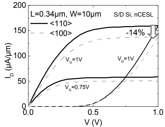
Figure II.43: I_D(V_G) et I_D(V_D) grille pour des nFET ( W=10 \mu\text{m} , L=0.34 \mu\text{m} ) sur SOI avec S/D Si et CESL neutre.
