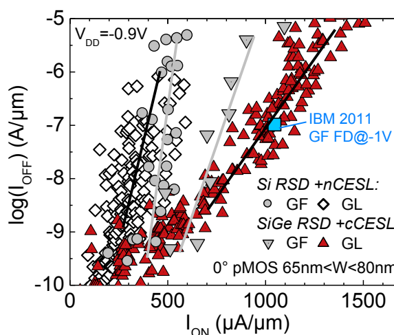
Figure III.39: I_{ON} - I_{OFF} de pFET FDSOI étroits avec une intégration gate-first et gate-last selon \langle 110 \rangle / (001) pour des configurations non contraintes et contraintes (S/D SiGe:B, cCESL).
