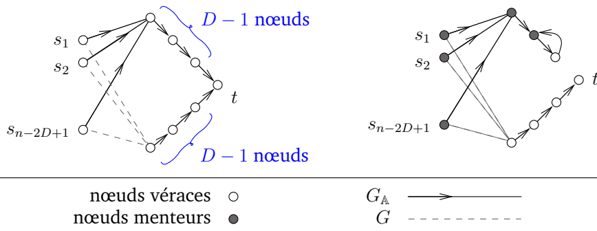
Figure 6.2: Un exemple de suppression d'arête conservant la connexité du graphe et créant n - (D + 1) menteurs dans un graphe de diamètre D .
