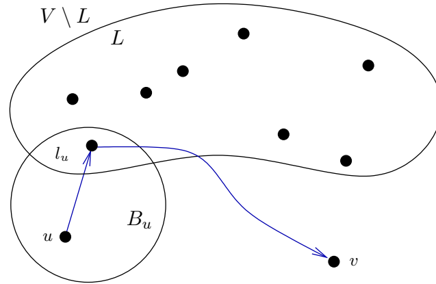
Figure 4.2: Routage du nœud u vers le nœud v avec l'algorithme LO
